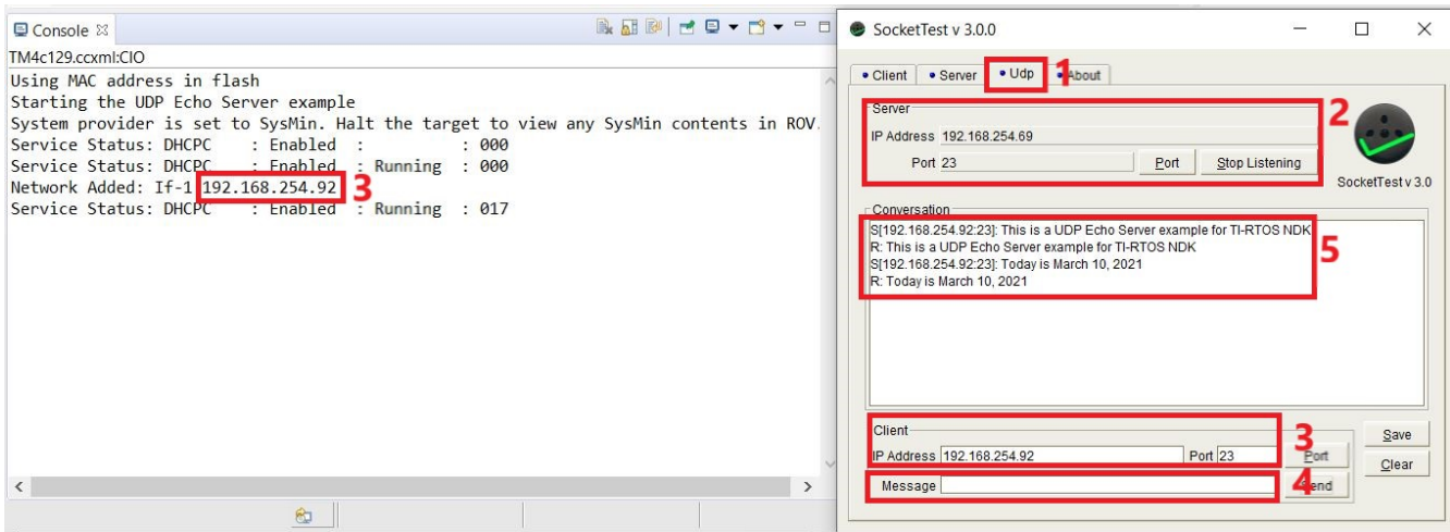
Figure 7-1. Enet_udpecho_server_tirtos Output
