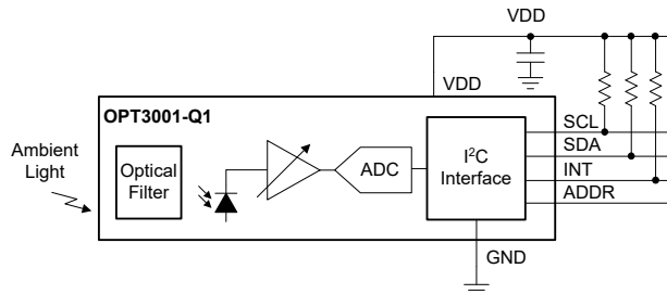
ブロック図
