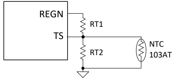
図 7-5. TS Pin Resistor Network
