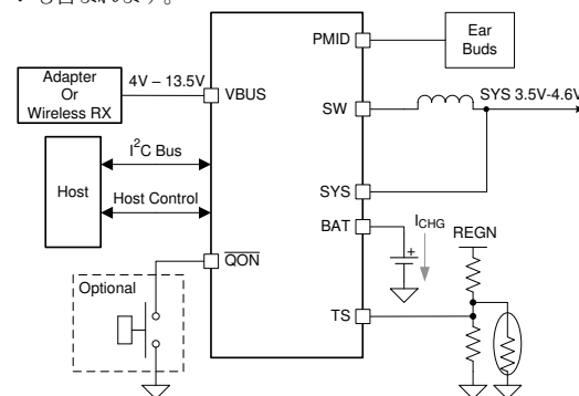
アプリケーション概略図
