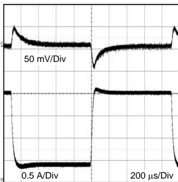
12 V_{IN} 3.3 V_O 0.6-A to 2-A Step
