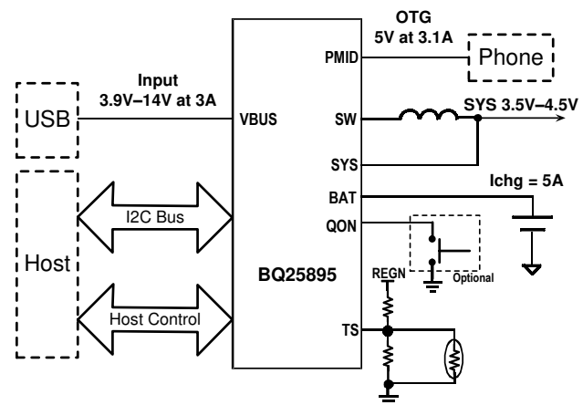
概略回路図
