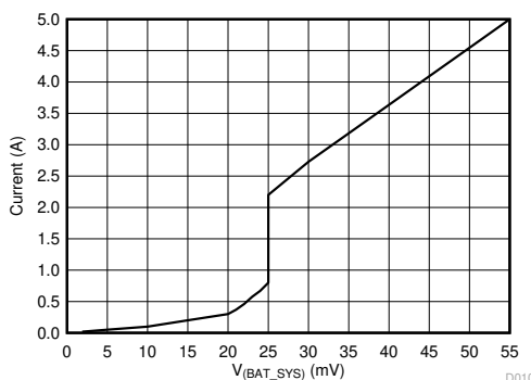
図 8-4. BATFET V-I Curve
