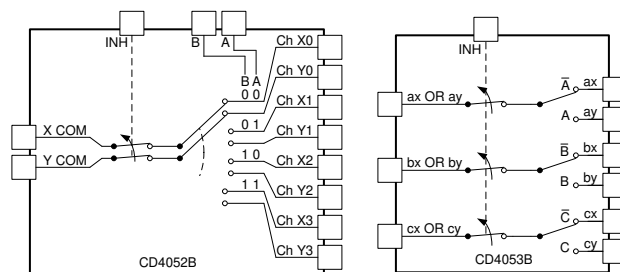
CD405xB の機能ブロック図
