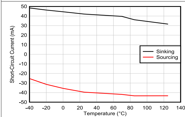
図 6-31. 短絡電流と温度との関係
