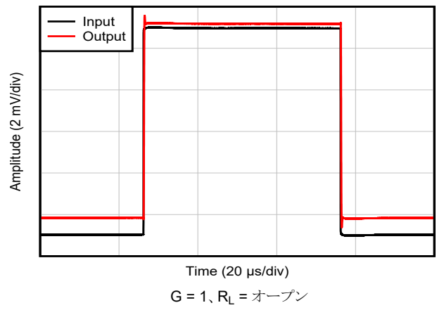
図 6-26. 小信号ステップ応答、 G = 1
