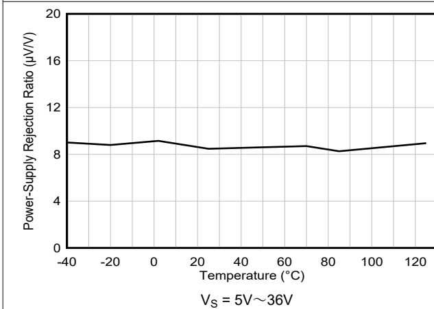
図 6-11. 電源除去比と温度との関係 (dB)
