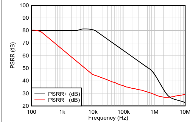
図 6-9. PSRR と周波数との関係
