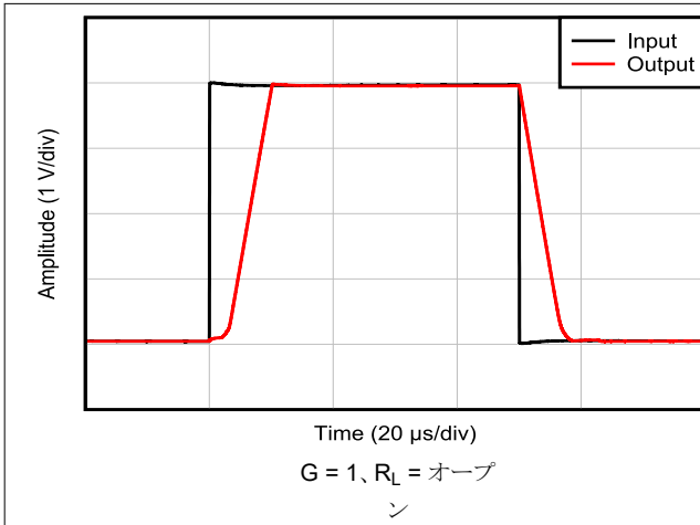
図 6-29. 大信号ステップ応答、 G = 1
