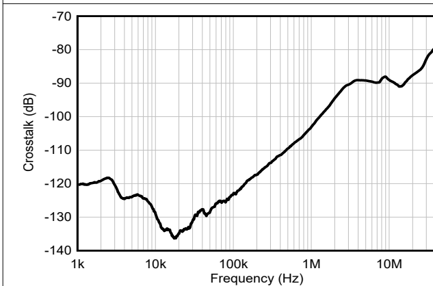
図 6-33. チャネル分離と周波数との関係
