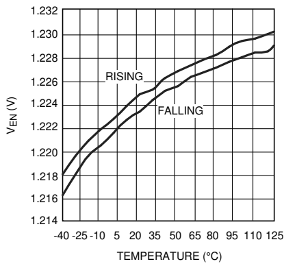
図 6-5. イネーブル・スレッシュヨルドと温度との関係
