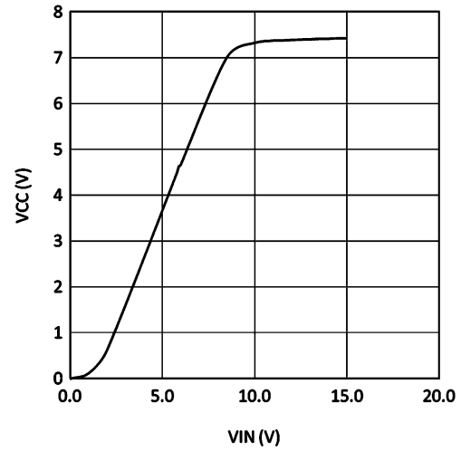
6-2. V_{CC} vs V_{IN}
