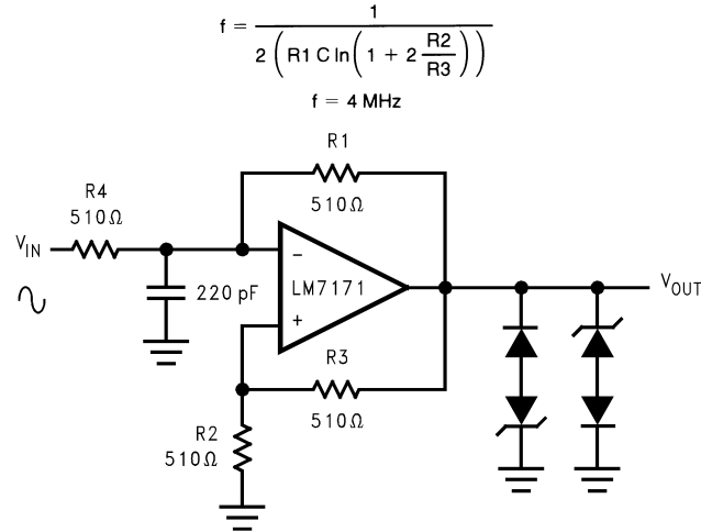
図 6-4. Pulse Width Modulator
