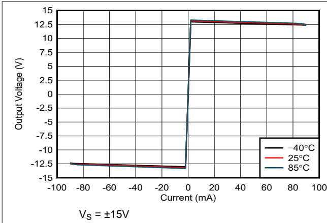
図 5-7. Output Voltage vs Output Current
