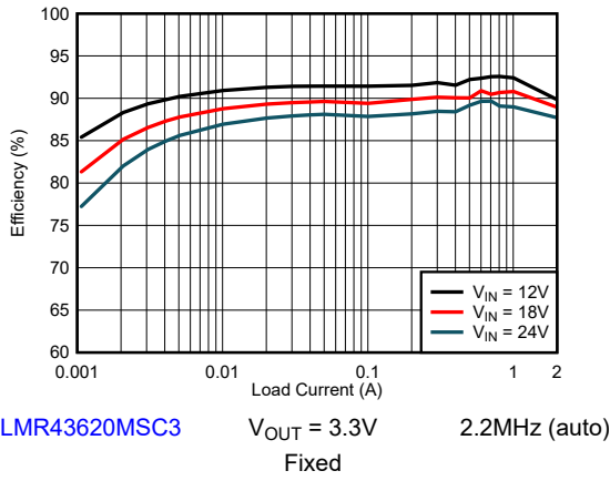
図 8-3. Efficiency
