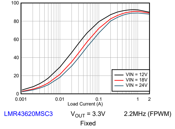
図 8-4. Efficiency
