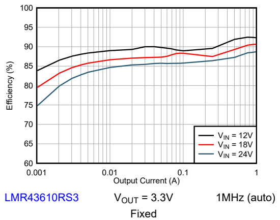
図 8-7. Efficiency
