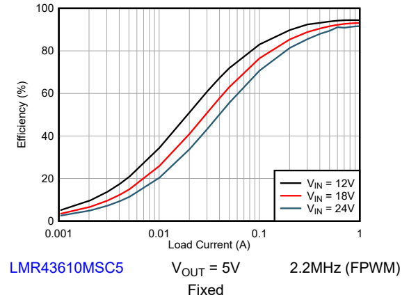
図 8-6. Efficiency
