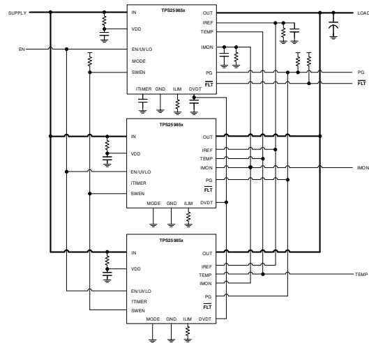
ブロック図
