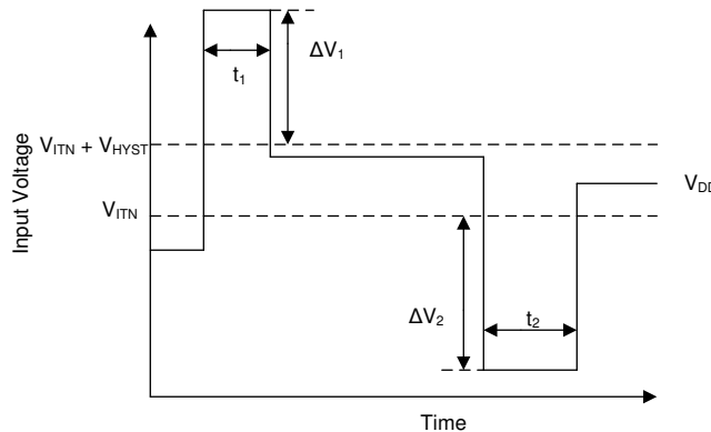
图 8-2. Overdrive Voltage
