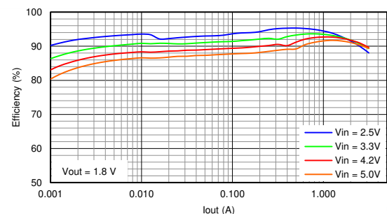
標準的なアプリケーションの効率
