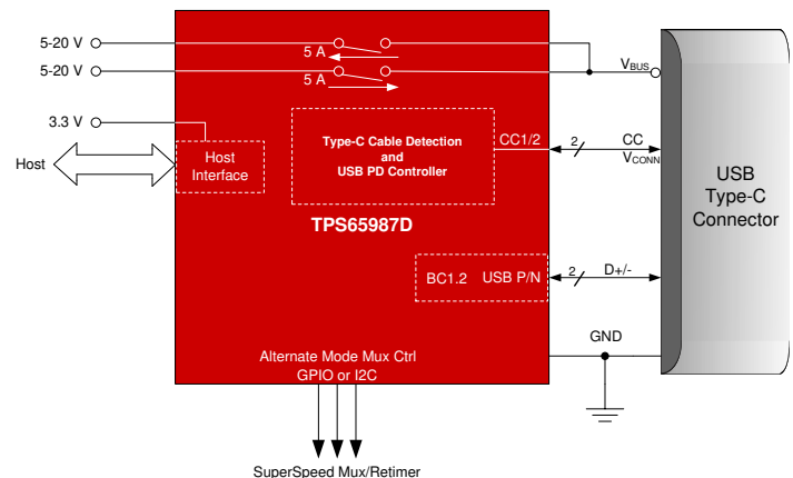
概略回路図
