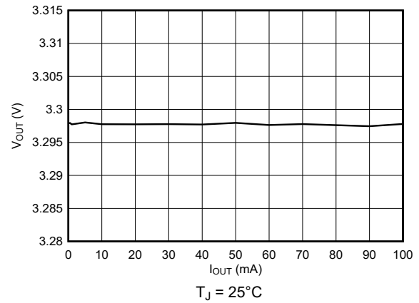
图 5-4. TPS76933-Q1 Output Voltage vs Output Current (New Chip)
