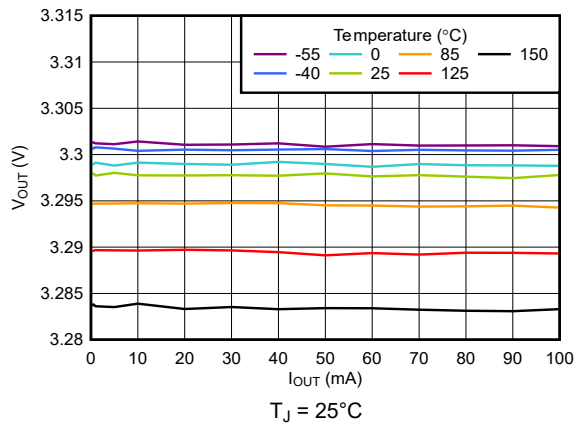
图 5-5. TPS76933-Q1 Output Voltage vs Output Current (New Chip)
