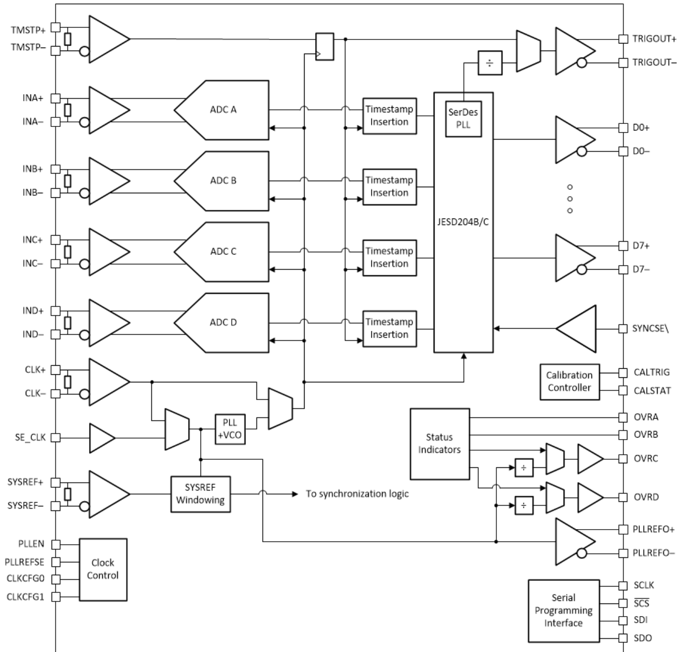
クワッドチャンネルのブロック図
