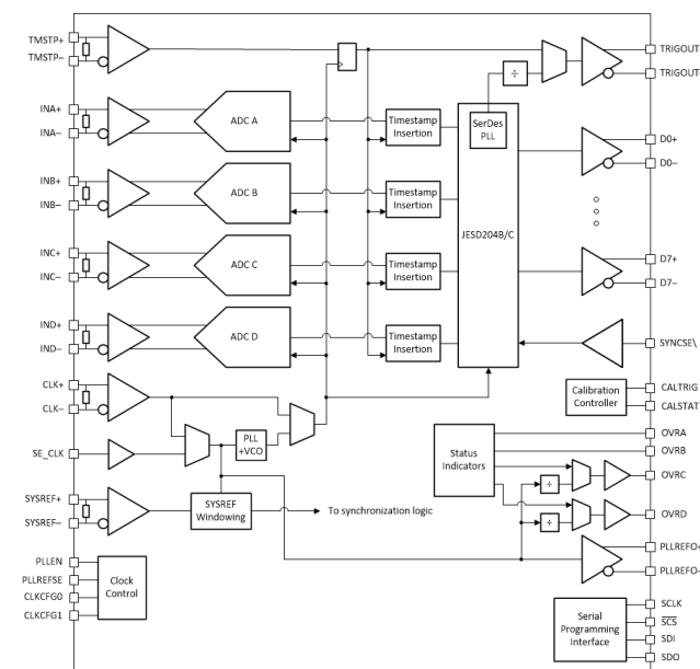
クワッド・チャンネルのブロック図
