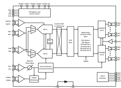
ADC12DJ5200RF ブロック図
