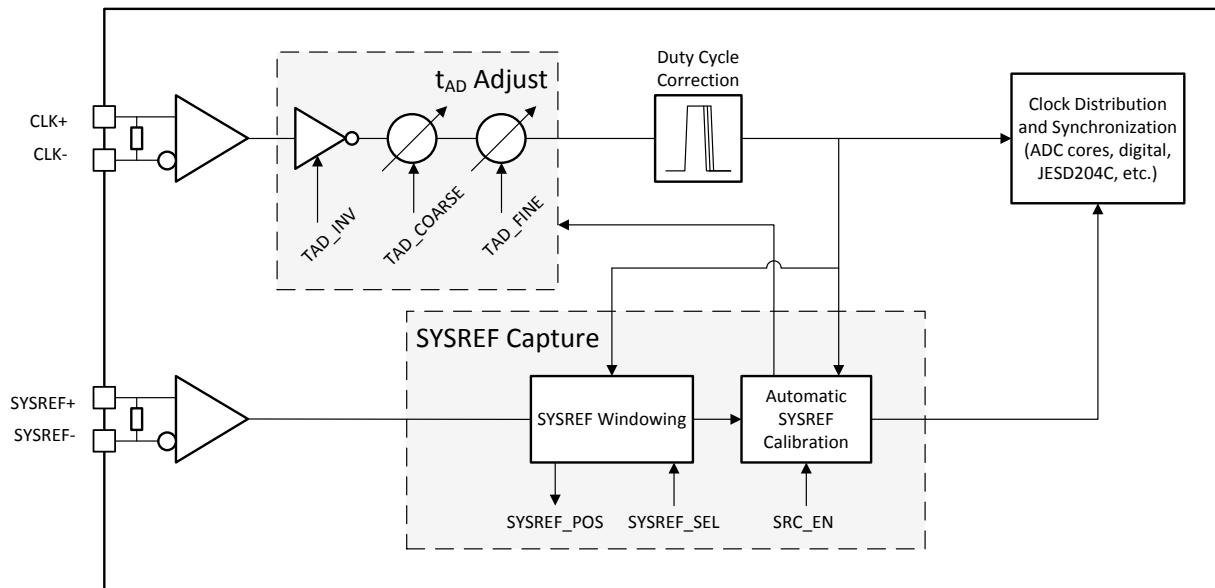
图 6-2. Clocking Subsystem
