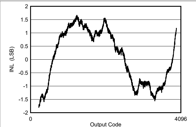
図 5-2. INL vs Code
