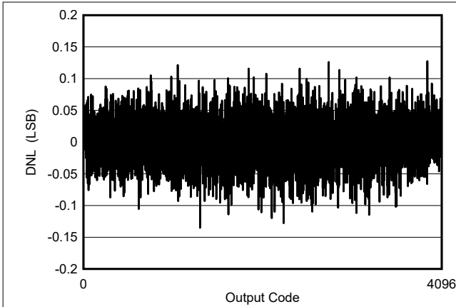
図 5-1. DNL vs Code
