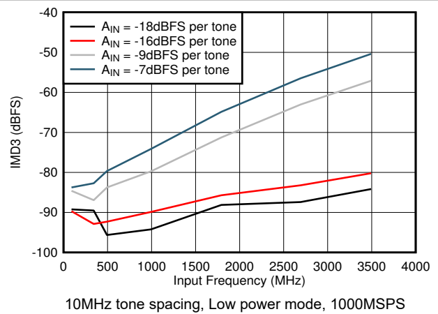
5-76. IMD3 vs F_{IN}
