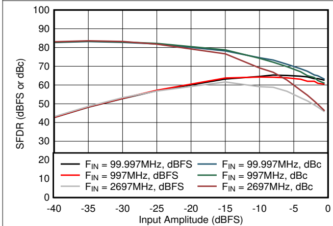
7-33. SFDR vs Input Amplitude
