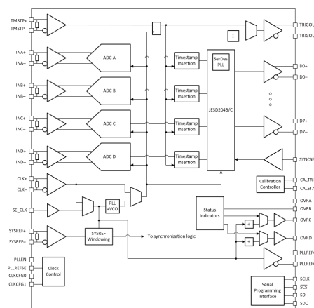
クワッド・チャンネルのブロック図
