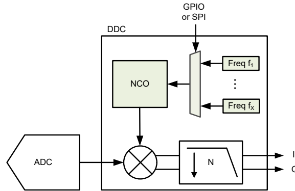
図 7-38. NCO Block Diagram
