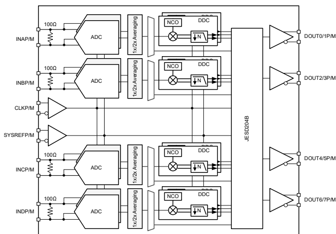
ブロック図
