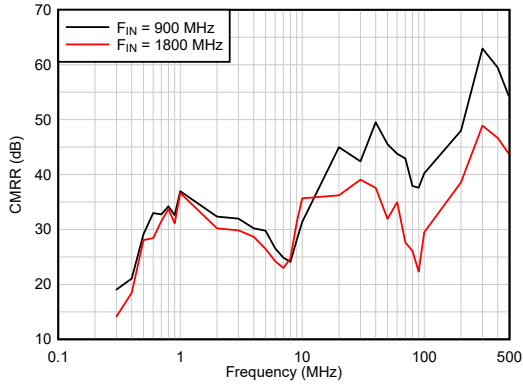
6-43. CMRR
