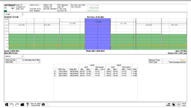
5-504. TX 100-MHz NR Output Spectrum at 4.9 GHz
