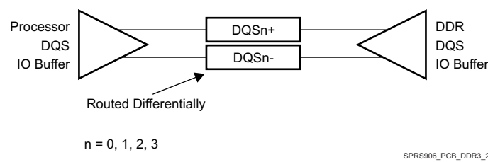
8-22. DQS Topology
