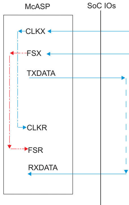
7-49. McASP1-8 CI-FI- - SYNC Mode
