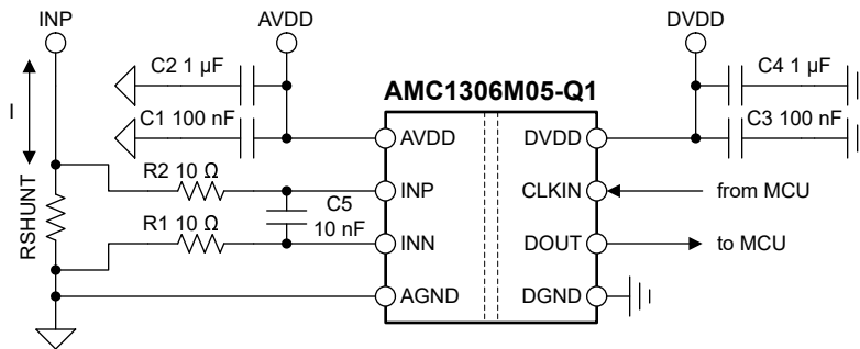
9-1. Decoupling of the AMC1306M05-Q1
