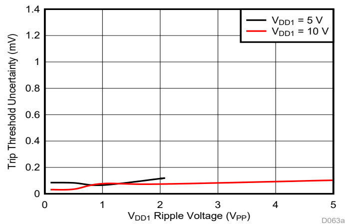
図 8-3. VDD1 リップル電圧に対するトリップ・スレッシュホールド感度 (f ripple = 10kHz)
