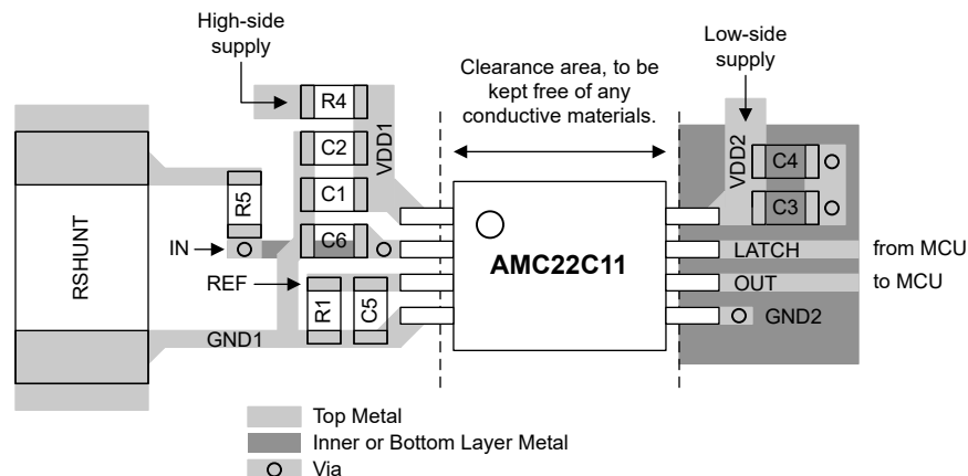
図 8-5. 推奨レイアウト： AMC22C11
