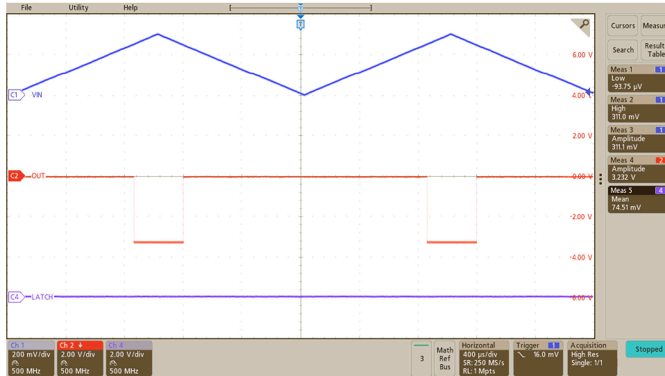
図 8-2. 三角入力波に対する AMC22C11 の出力応答
