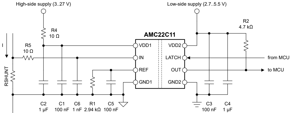
図 8-4. デカップリング： AMC22C11
