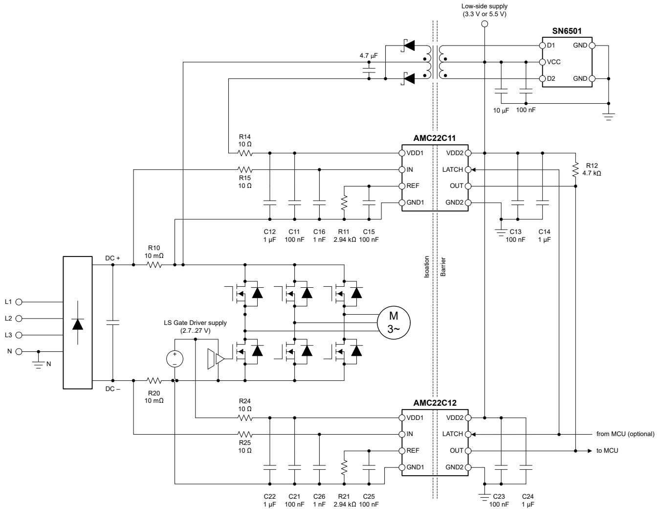
図 8-1. AMC22C11 による DC+ 過電流検出
