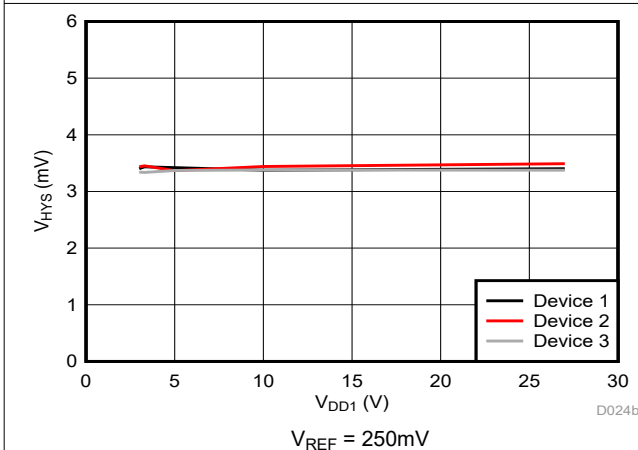
図 6-15. のトリップ・スレッシュホールドのヒステリシスと電源電圧との関係
