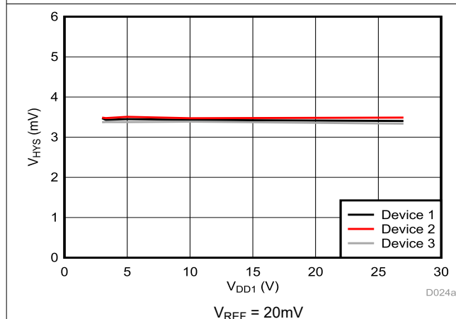
図 6-9. のトリップ・スレッシュホールドのヒステリシスと電源電圧との関係
