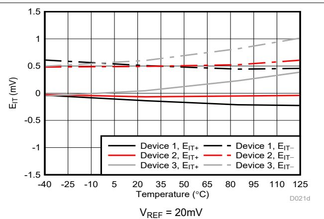
図 6-8. のトリップ・スレッシュホールド誤差と温度との関係
