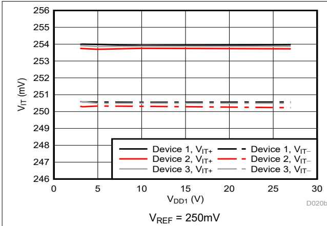
図 6-11. のトリップ・スレッシュولدと電源電圧との関係
