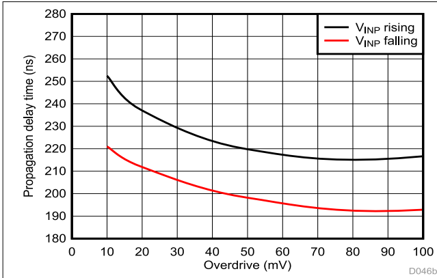
図 6-23. 伝搬遅延とオーバードライブとの関係
