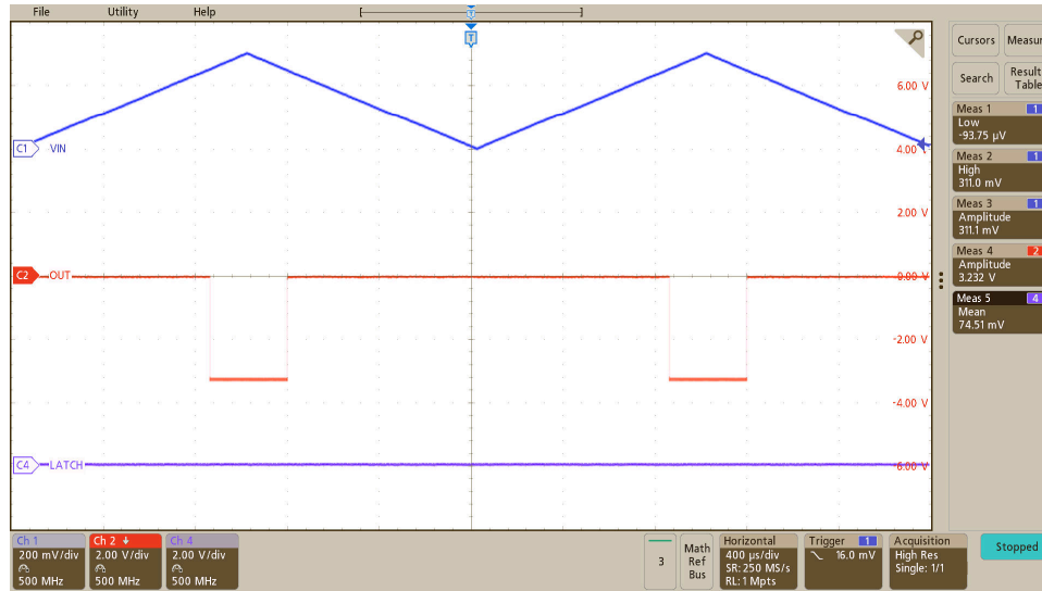
図 8-2. 三角入力波に対する AMC22C11-Q1 の出力応答
