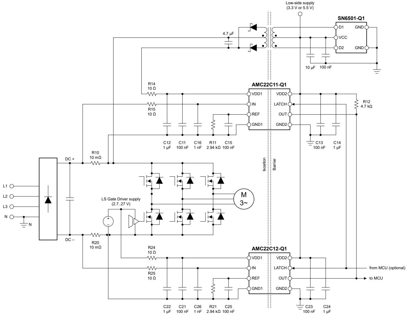
図 8-1. AMC22C11-Q1 による DC+ 過電流検出
