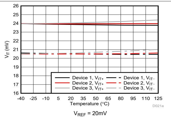
図 6-6. のトリップ・スレッシュホールドと温度との関係
