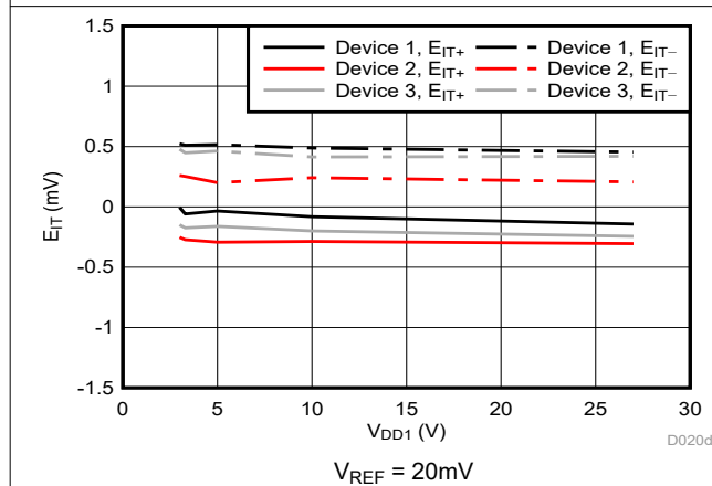
図 6-7. のトリップ・スレッシュホールド誤差と電源電圧との関係
