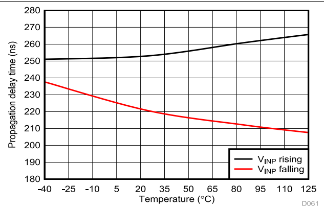
図 6-24. 伝搬遅延と温度との関係
