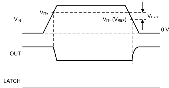
図 7-1. スwitchング・スレッシュホールドとヒステリシス
