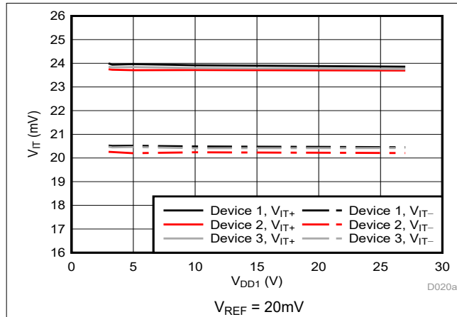
図 6-5. のトリップ・スレッシュホールドと電源電圧との関係
