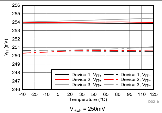
図 6-12. のトリップ・スレッシュولدと温度との関係
