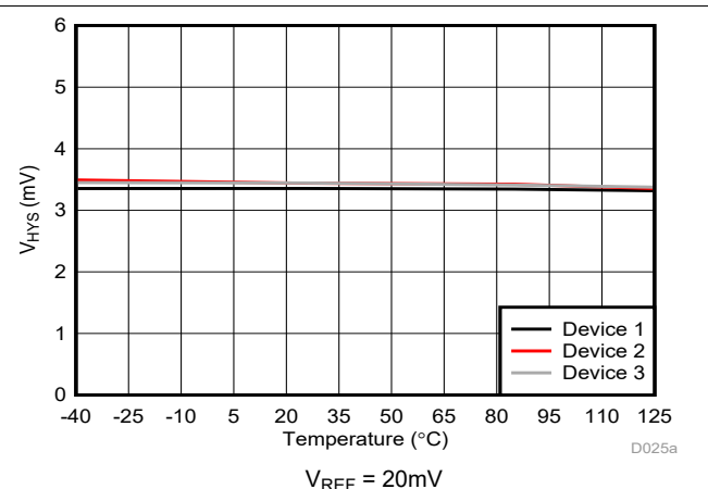
図 6-10. のトリップ・スレッシュホールドのヒステリシスと温度との関係
