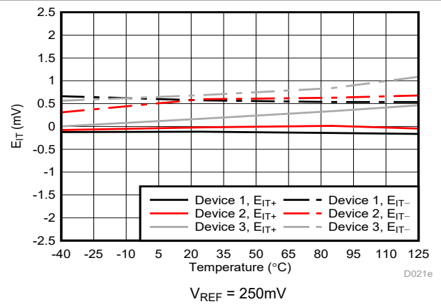
図 6-14. のトリップ・スレッシュولد誤差と温度との関係
