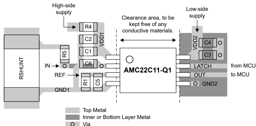
図 8-5. 推奨レイアウト： AMC22C11-Q1
