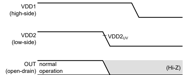
図 7-10. VDD2 がオフになってから VDD1 がオフになる
