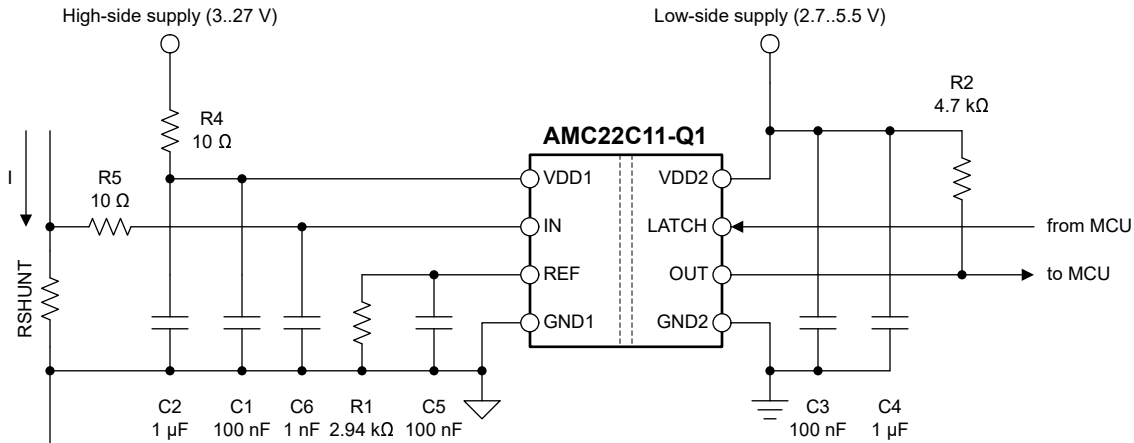
図 8-4. デカップリング： AMC22C11-Q1
