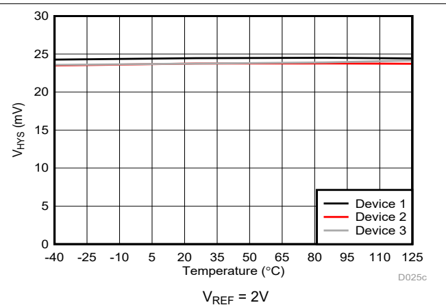
図 6-22. のトリップ・スレッシュホールドのヒステリシスと温度との関係
