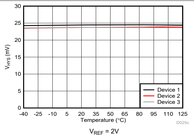
図 6-22. Cmp0 のトリップ・スレッシュールドのヒステリシスと温度との関係
