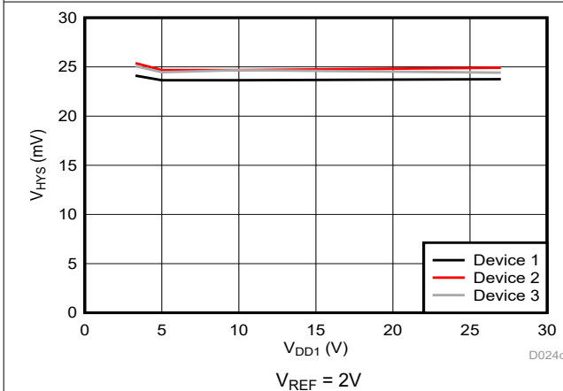
図 6-21. Cmp0 のトリップ・スレッシュールドのヒステリシスと電源電圧との関係
