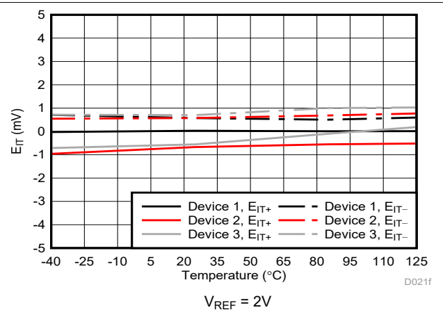
図 6-20. Cmp0 のトリップ・スレッシュールド誤差と温度との関係
