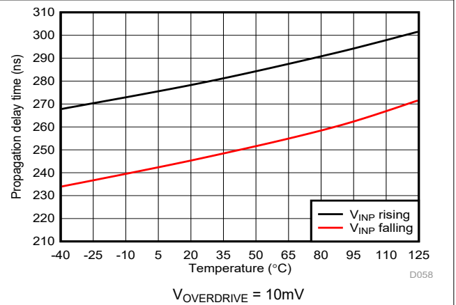
図 6-38. Cmp1 の伝搬遅延と温度との関係
