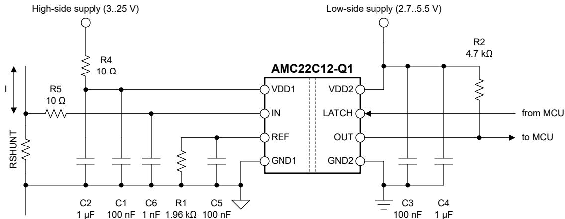
図 8-6. デカップリング：AMC22C12-Q1
