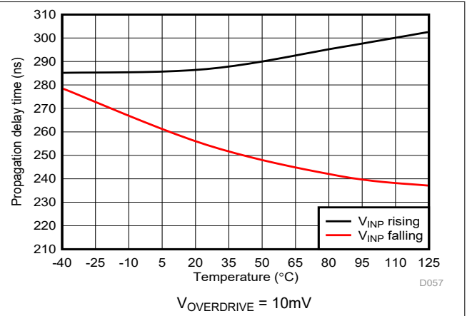
図 6-36. Cmp0 の伝搬遅延と温度との関係
