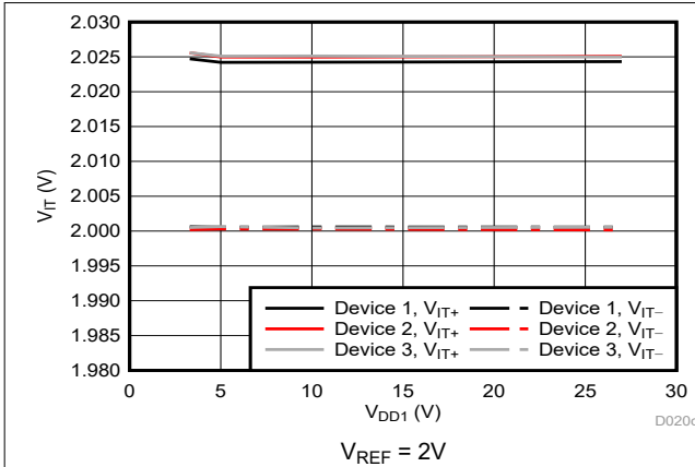
図 6-17. Cmp0 のトリップ・スレッシュールドと電源電圧との関係
