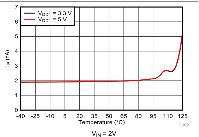
図 6-40. の入力バイアス電流と温度との関係
