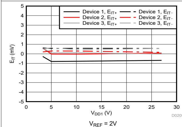
図 6-19. Cmp0 のトリップ・スレッシュールド誤差と電源電圧との関係
