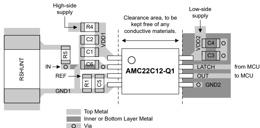
図 8-7. 推奨レイアウト：AMC22C12-Q1
