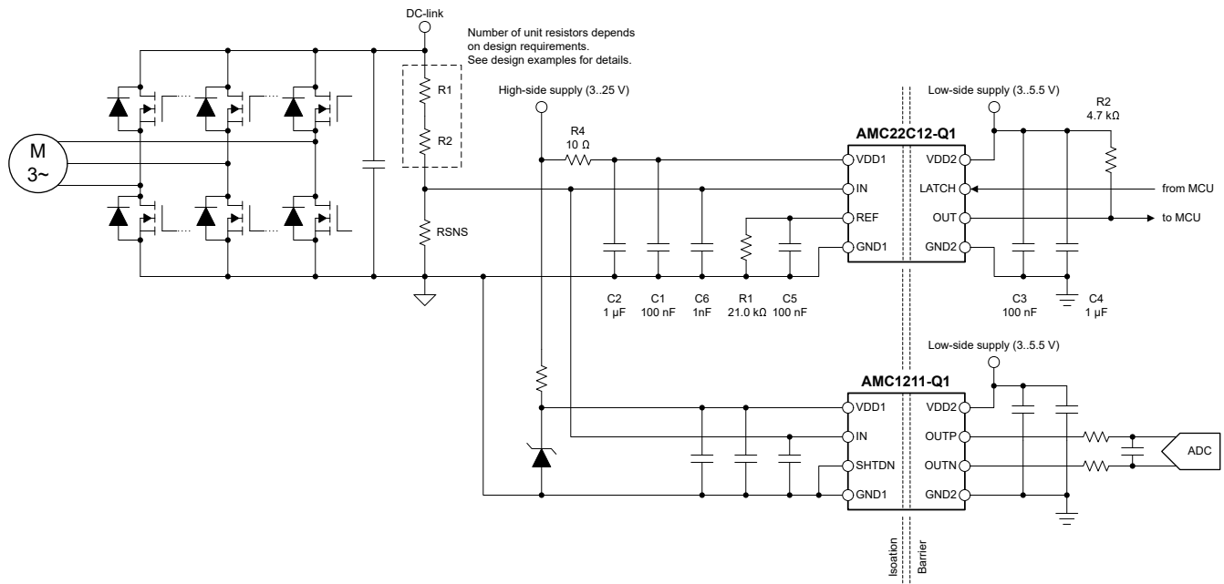
図 8-2. AMC22C12-Q1 による過電圧検出
