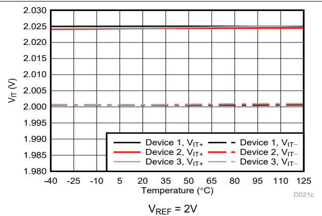
図 6-18. Cmp0 のトリップ・スレッシュールドと温度との関係
