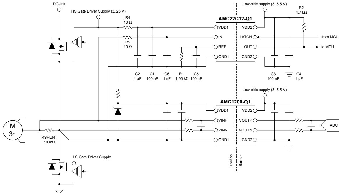
図 8-1. AMC22C12-Q1 による過電流の検出
