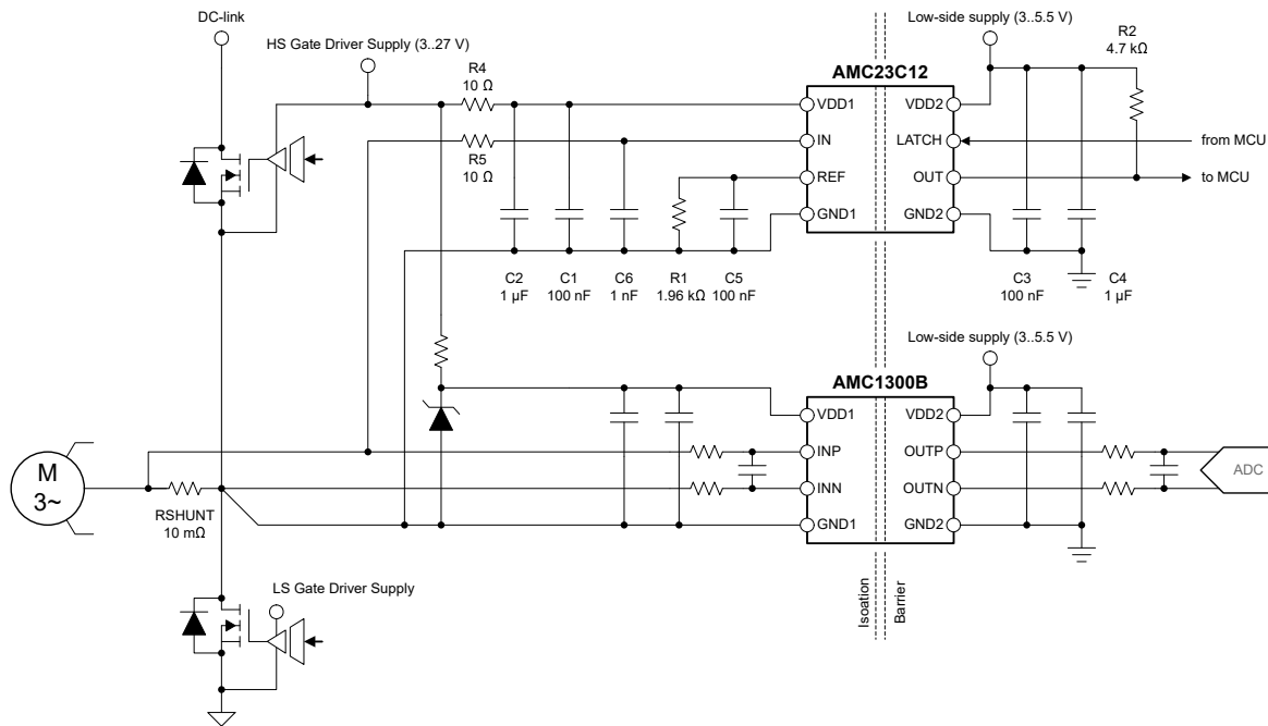
図 8-1. AMC23C12 による過電流の検出
