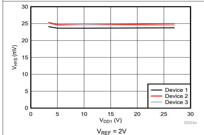
図 6-21. Cmp0 のトリップ・スレッシュホールドのヒステリシスと電源電圧との関係
