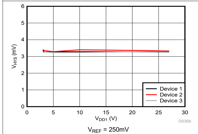
図 6-33. Cmp1 のトリップ・スレッショルドのヒステリシスと電源電圧との関係
