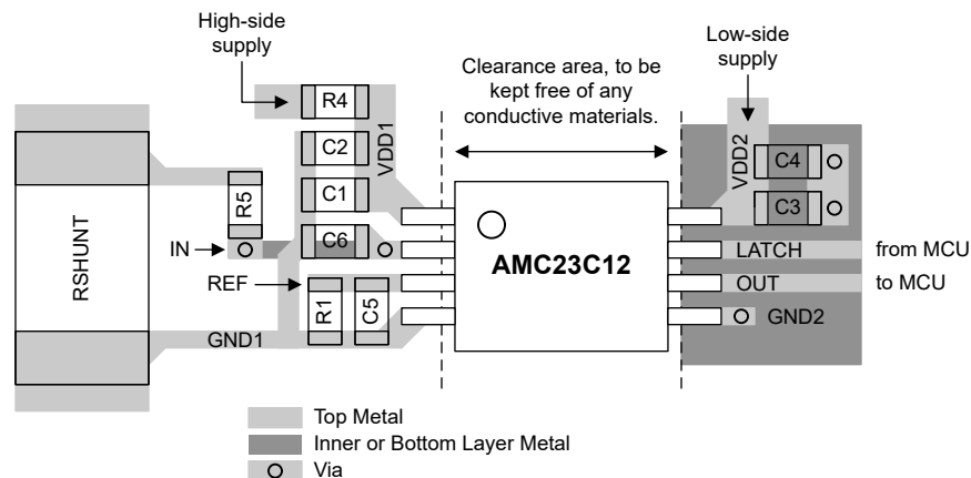
図 8-7. 推奨レイアウト：AMC23C12
