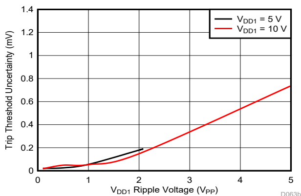
図 8-5. VDD1 リップル電圧に対するトリップ・スレッシュホールド感度 (Cmp1、 f_{RIPPLE} = 10\text{kHz} )
