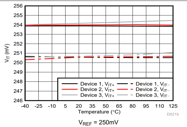
図 6-12. Cmp0 のトリップ・スレッシュヨルドと温度との関係
