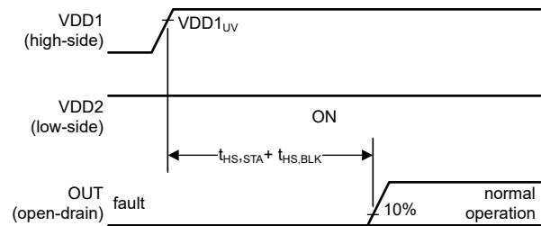
図 7-6. VDD2 はオン、VDD1 がオンする (長い遅延)
