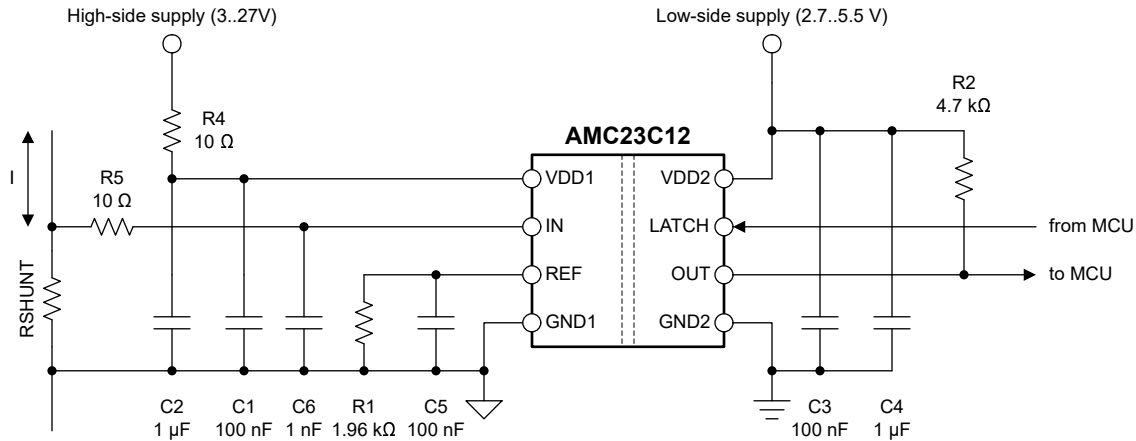
図 8-6. デカップリング：AMC23C12
