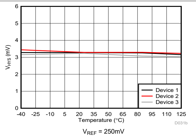
図 6-34. Cmp1 のトリップ・スレッショルドのヒステリシスと温度との関係
