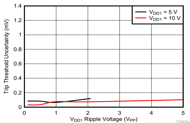
図 8-4. VDD1 リップル電圧に対するトリップ・スレッシュホールド感度 (Cmp0、 f_{RIPPLE} = 10\text{kHz} )
