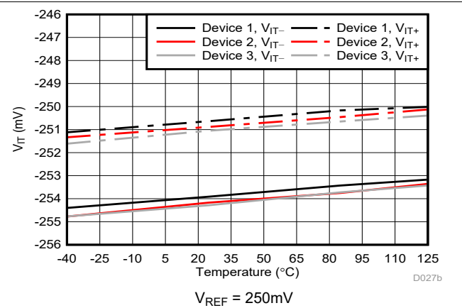
図 6-30. Cmp1 のトリップ・スレッショルドと温度との関係
