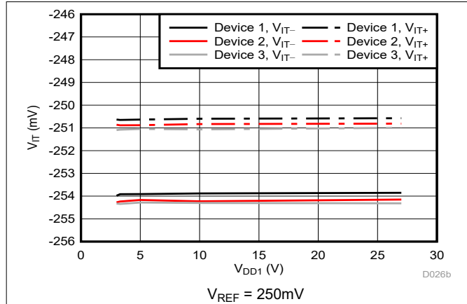
図 6-29. Cmp1 のトリップ・スレッショルドと電源電圧との関係
