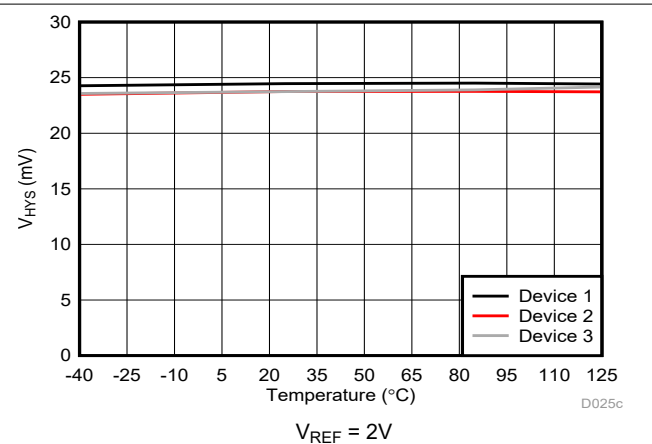
図 6-22. Cmp0 のトリップ・スレッシュホールドのヒステリシスと温度との関係
