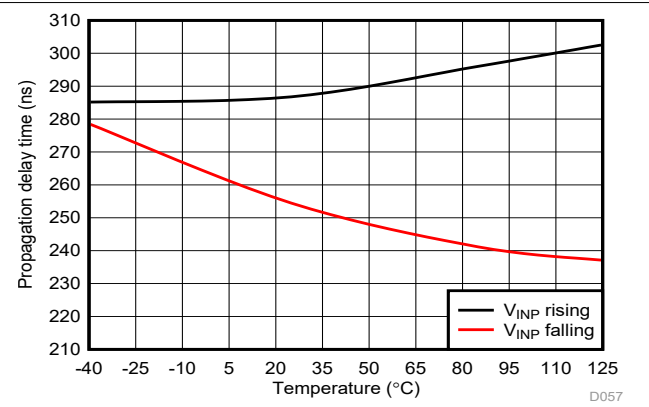
図 6-36. Cmp0 の伝搬遅延と温度との関係
