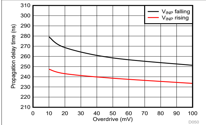
図 6-35. Cmp0 の伝搬遅延とオーバードライブとの関係
