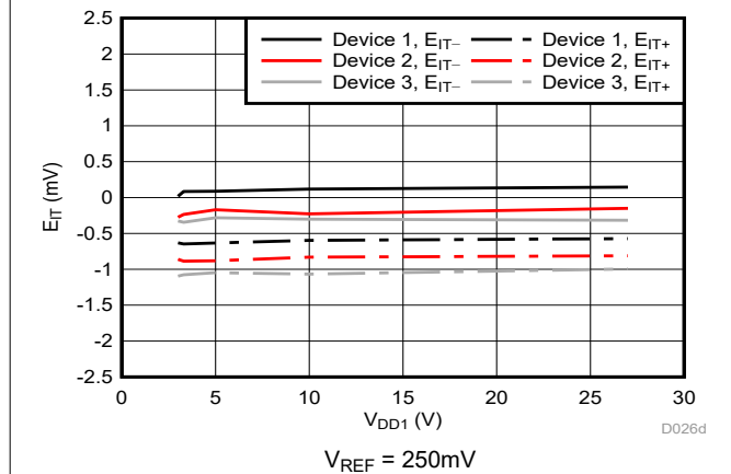
図 6-31. Cmp1 のトリップ・スレッショルド誤差と電源電圧との関係
