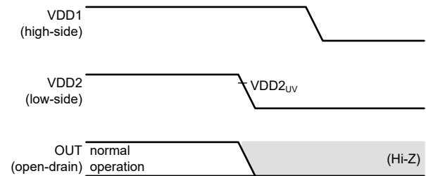
図 7-10. VDD2 がオフし、VDD1 がそれに続く
