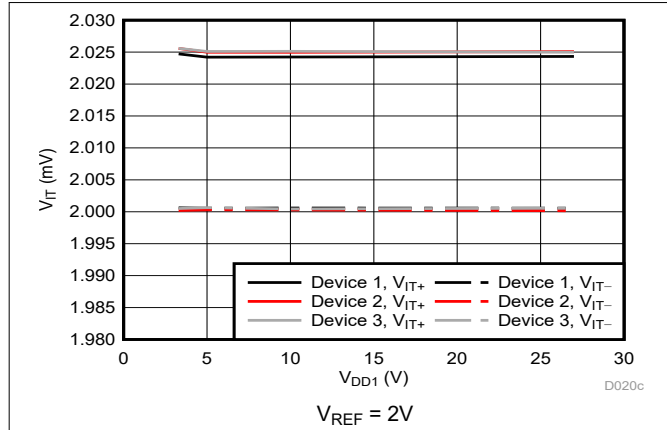
図 6-17. Cmp0 のトリップ・スレッシュホールドと電源電圧との関係
