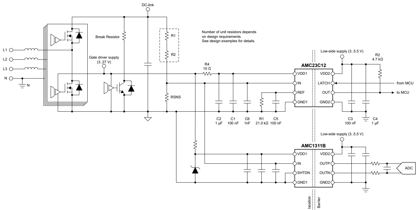
図 8-2. AMC23C12 による過電圧検出
