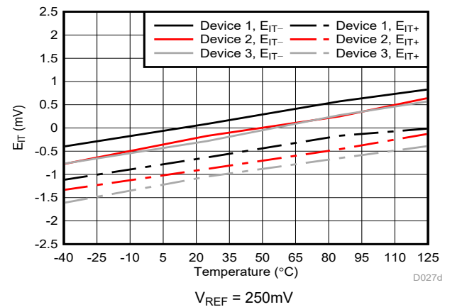
図 6-32. Cmp1 のトリップ・スレッショルド誤差と温度との関係
