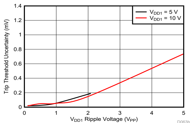
図 8-5. VDD1 リップル電圧に対するトリップ・スレッシュホールド感度 (Cmp1、 f_{\text{RIPPLE}} = 10\text{kHz} )
