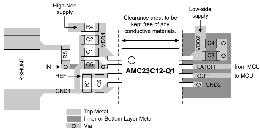
図 8-7. 推奨レイアウト：AMC23C12-Q1
