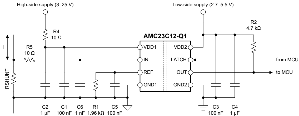
図 8-6. デカップリング：AMC23C12-Q1
