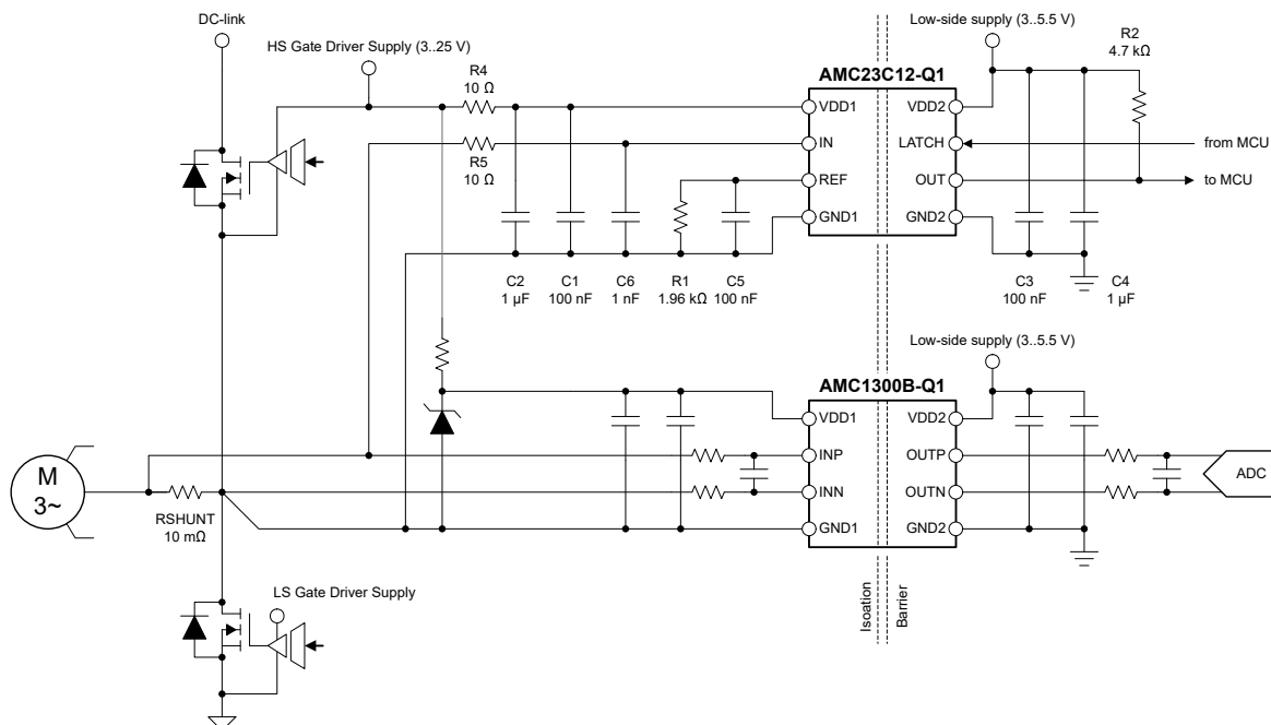
図 8-1. AMC23C12-Q1 による過電流の検出
