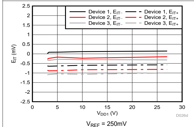
図 6-31. Cmp1 のトリップ・スレッショルド誤差と電源電圧との関係
