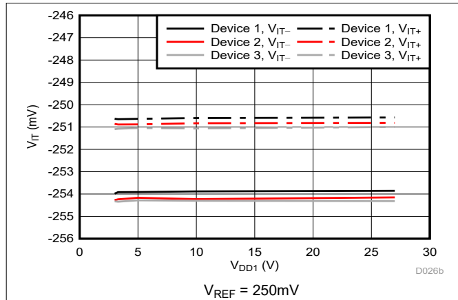
図 6-29. Cmp1 のトリップ・スレッショルドと電源電圧との関係
