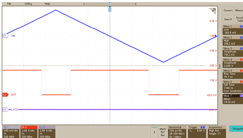
図 8-3. 三角入力波に対する AMC23C12-Q1 の出力応答
