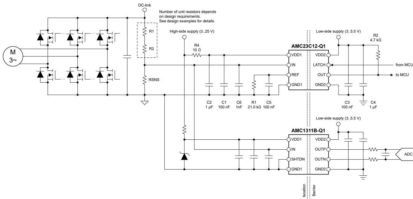
図 8-2. AMC23C12-Q1 による過電圧検出
