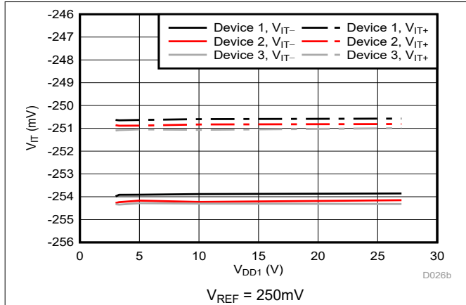
図 6-41. Cmp1 のトリップ・スレッシュホールドと電源電圧との関係
