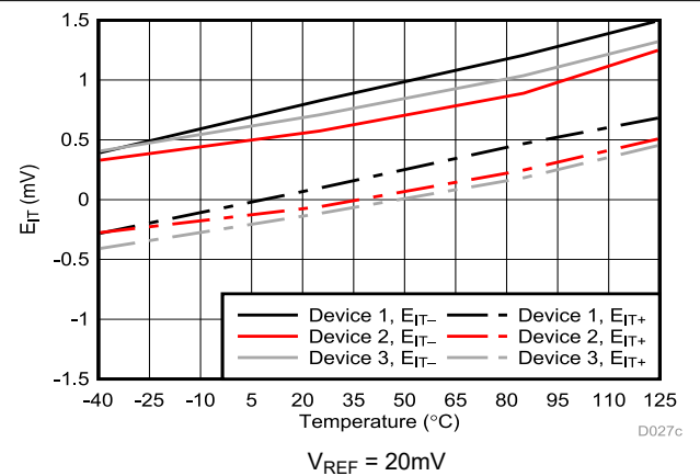
図 6-38. Cmp1 のトリップ・スレッシュォルド誤差と温度との関係
