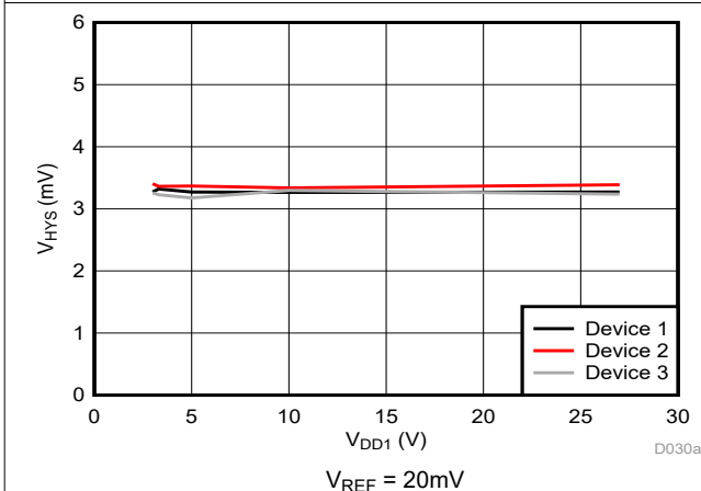
図 6-39. Cmp1 のトリップ・スレッシュォルドのヒステリシスと電源電圧との関係
