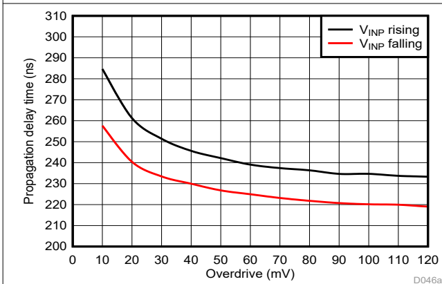
図 6-49. Cmp3 の伝搬遅延とオーバードライブとの関係
