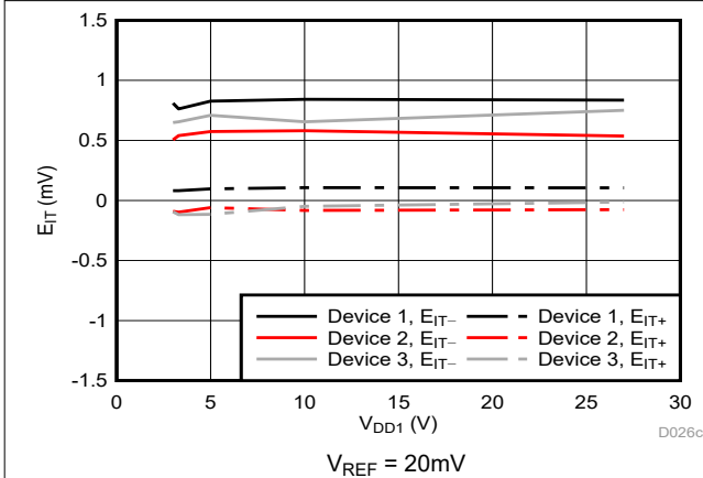
図 6-37. Cmp1 のトリップ・スレッシュォルド誤差と電源電圧との関係
