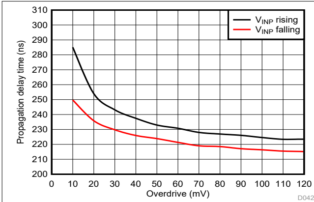
図 6-47. Cmp2 の伝搬遅延とオーバードライブとの関係
