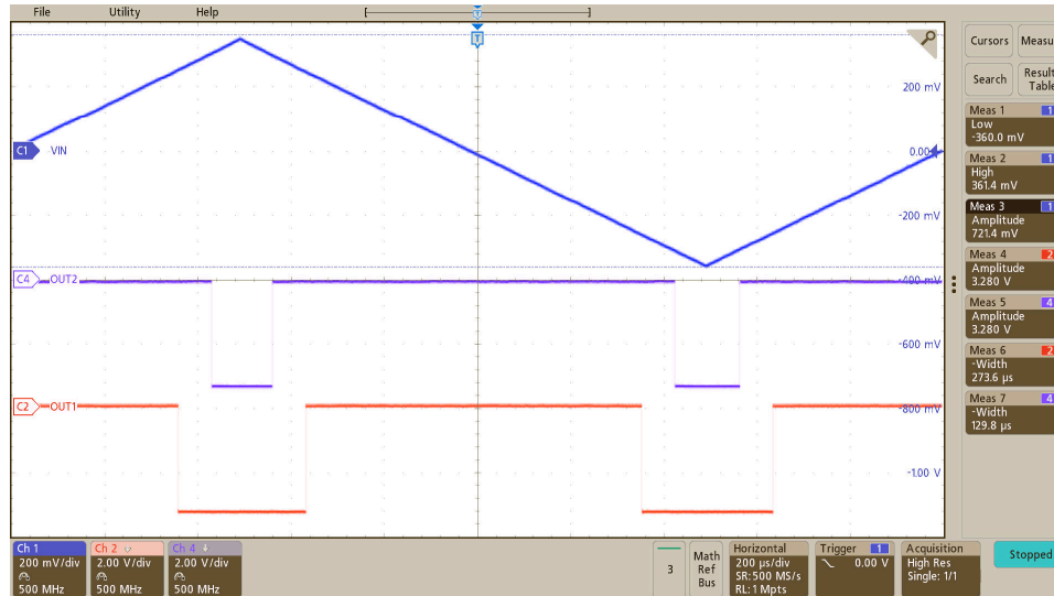
図 8-2. 三角入力波に対する AMC23C15 の出力応答
