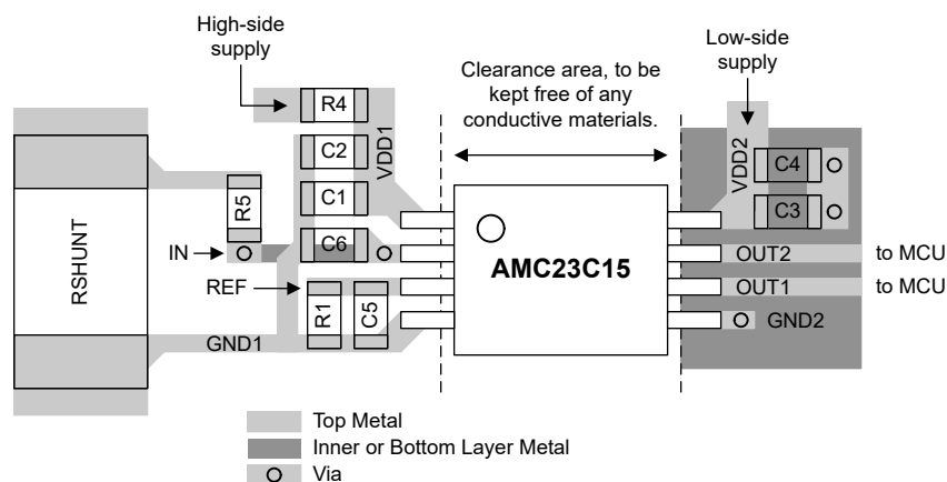
図 8-8. 推奨レイアウト：AMC23C15
