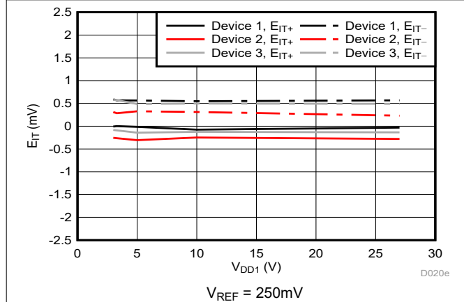
図 6-25. Cmp0 のトリップ・スレッシュヨルド誤差と電源電圧との関係
