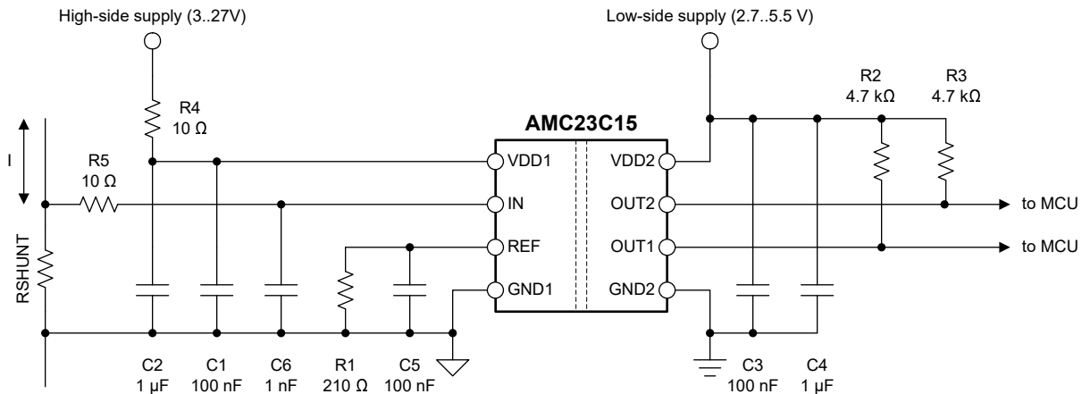
図 8-7. デカップリング：AMC23C15
