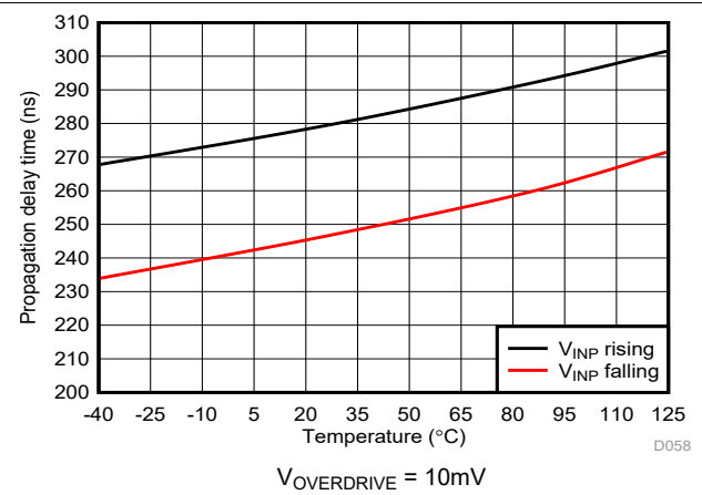
図 6-54. Cmp1 の伝搬遅延と温度との関係
