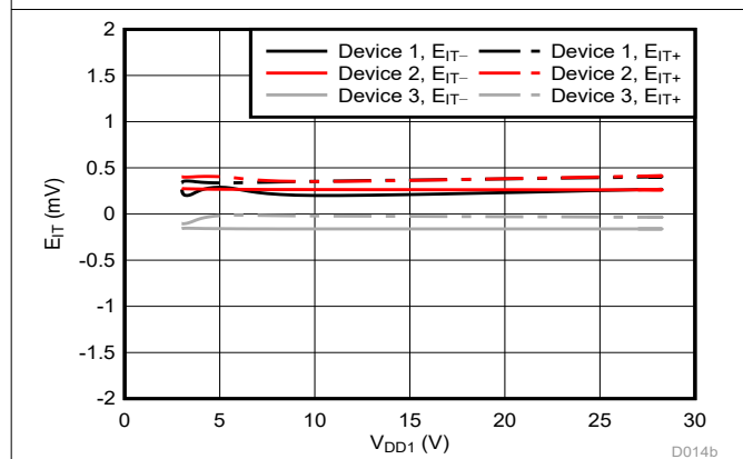
図 6-11. Cmp3 のトリップ・スレッシュォルドと電源電圧との関係
