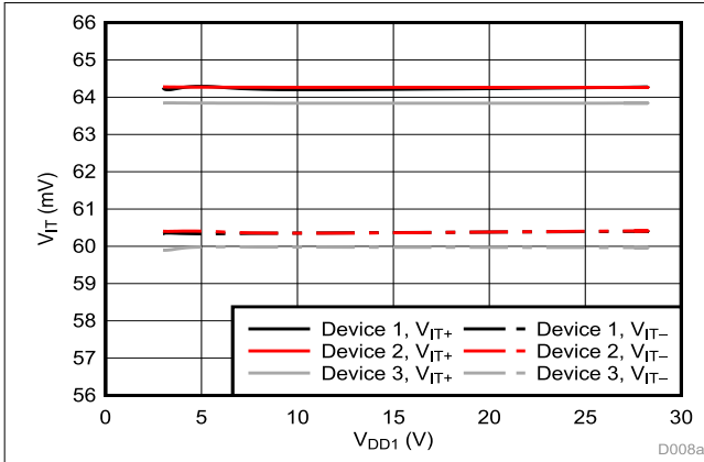
図 6-5. Cmp2 のトリップ・スレッシュホールドと電源電圧との関係
