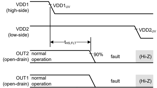
図 7-8. VDD1 がオフになってから VDD2 がオフになる
