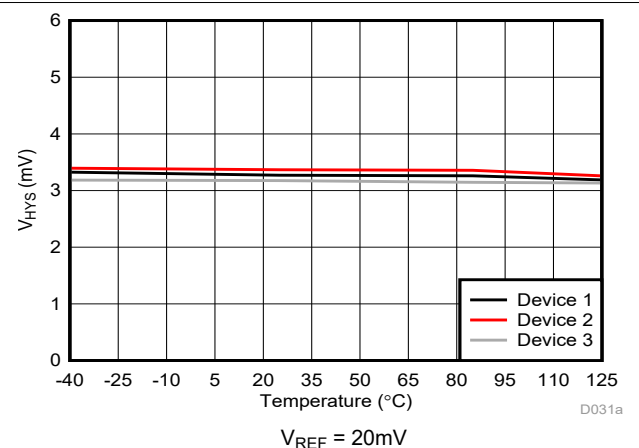
図 6-40. Cmp1 のトリップ・スレッシュォルドのヒステリシスと温度との関係
