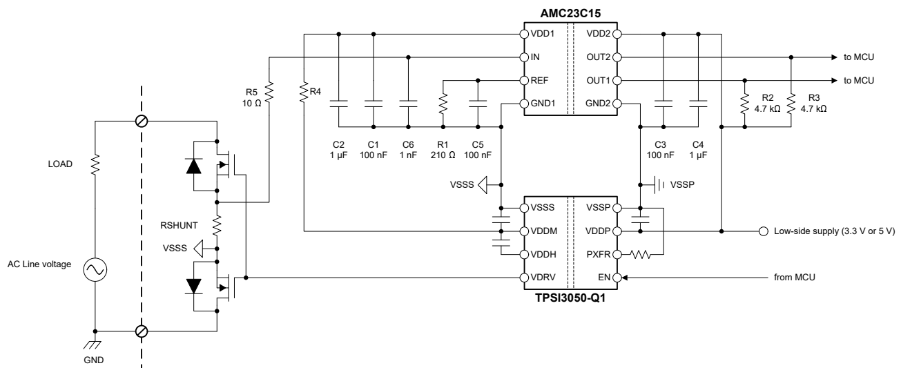
図 8-1. AMC23C15 による過電流および短絡の検出
