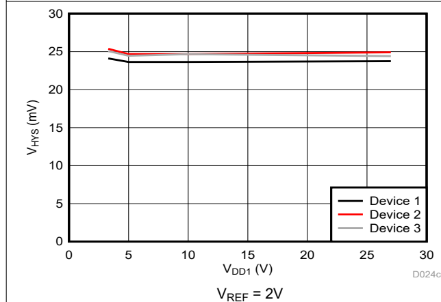
図 6-33. Cmp0 のトリップ・スレッシュホールドのヒステリシスと電源電圧との関係
