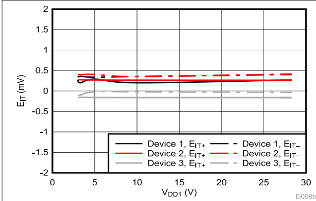
図 6-5. Cmp2 のトリップ・スレッシュホールドと電源電圧との関係
