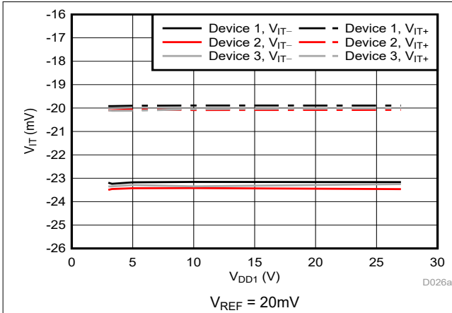
図 6-35. Cmp1 のトリップ・スレッシュォルドと電源電圧との関係
