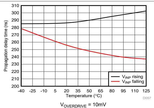
図 6-52. Cmp0 の伝搬遅延と温度との関係
