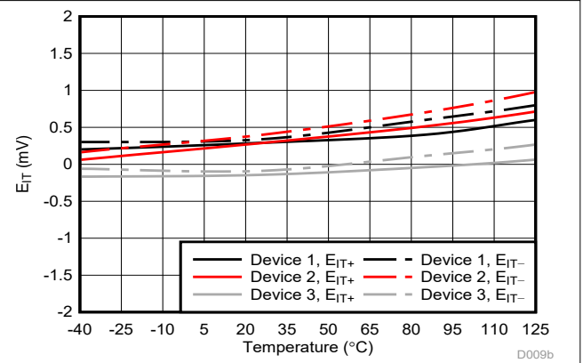
図 6-6. Cmp2 のトリップ・スレッシュホールドと温度との関係
