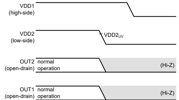
図 7-10. VDD2 がオフになってから VDD1 がオフになる
