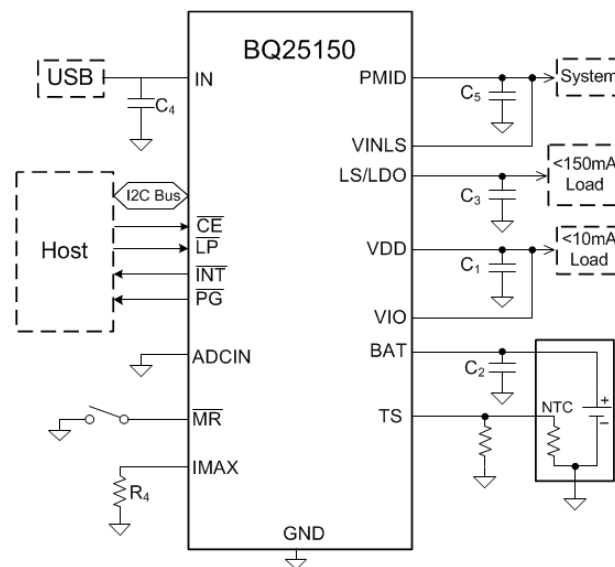
簡略回路図
