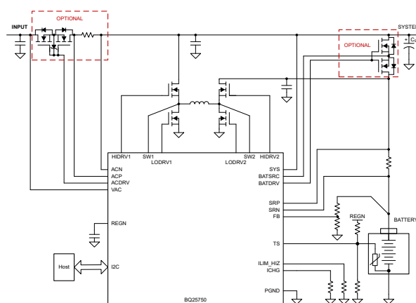
概略回路図
