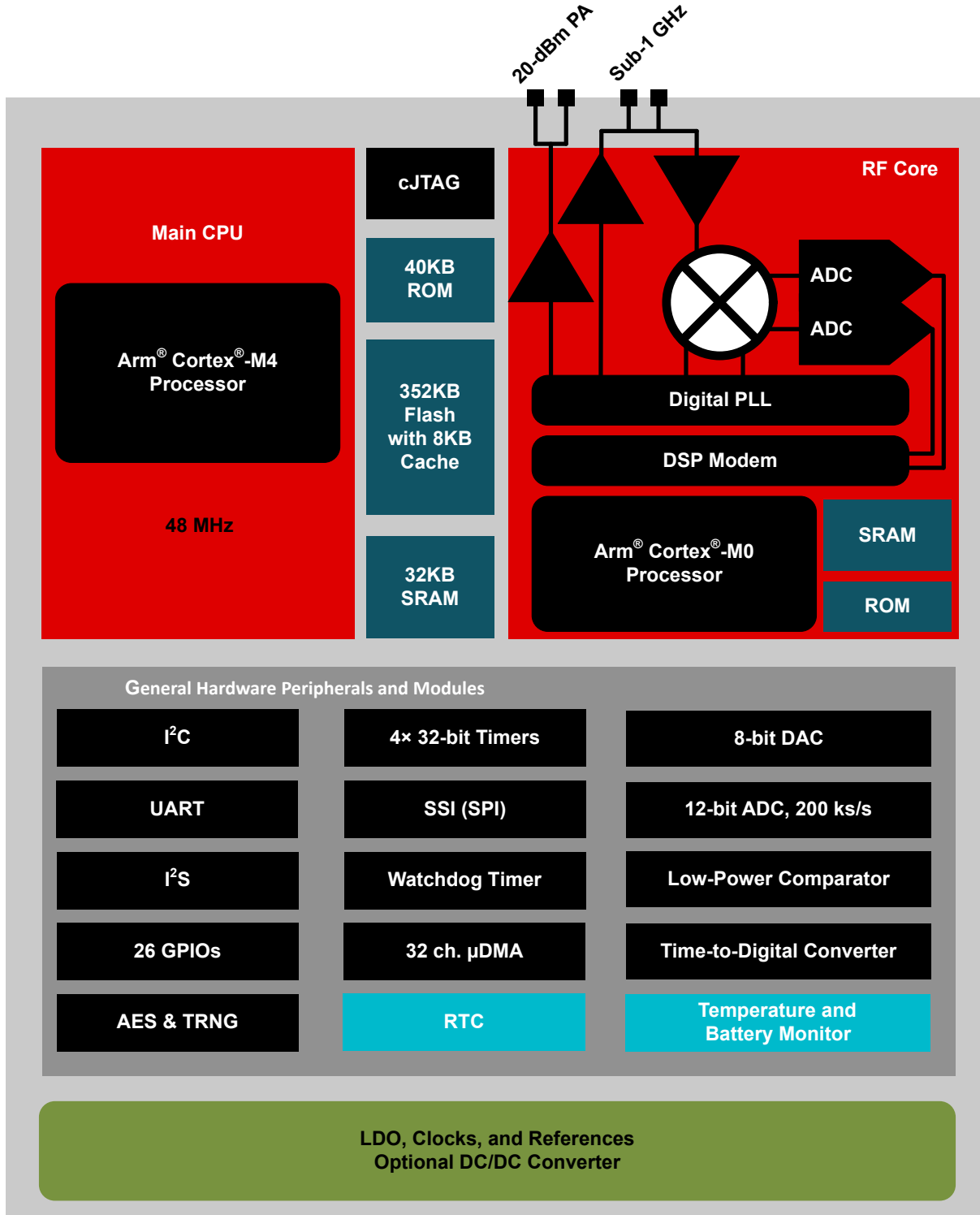
図 4-1. CC1311P3 機能ブロック図
