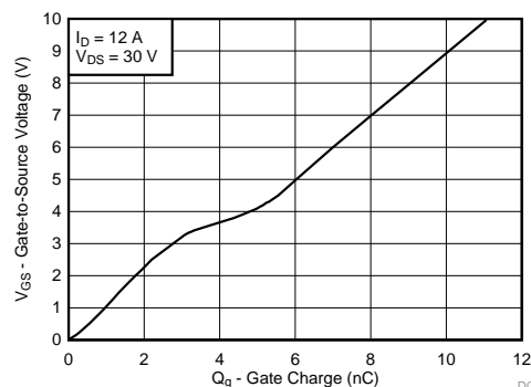
ゲート電荷
