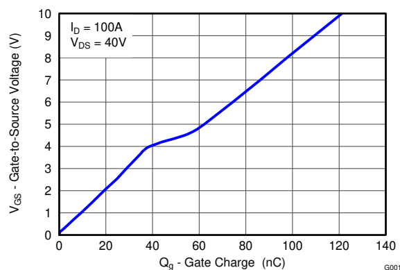
ゲート電荷
