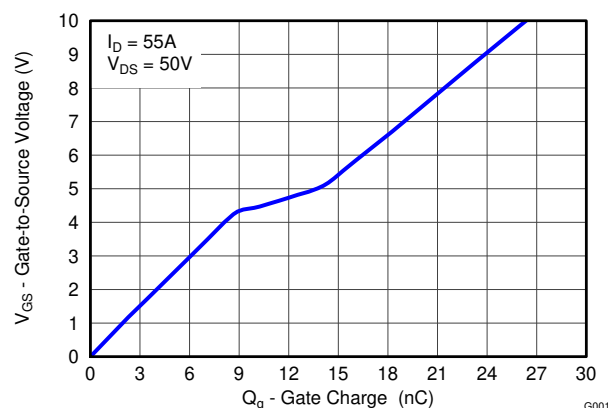
ゲート電荷
