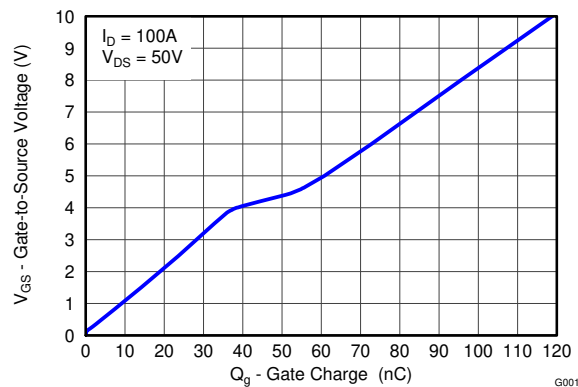
ゲート電荷
