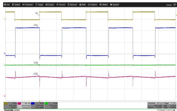
A. チャンネル 1 = IN1 チャンネル 2 = モーター電流 チャンネル 3 = OUT1 チャンネル 4 = OUT2
