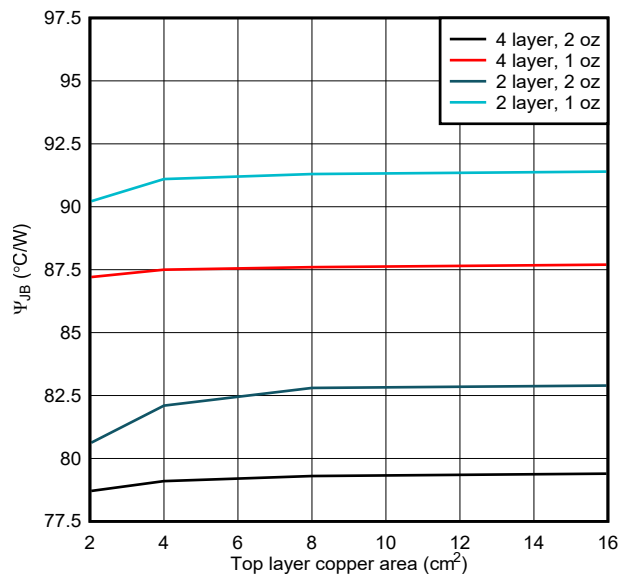
図 9-31. SOT、接合部から基板への特長パラメータと銅面積との関係
