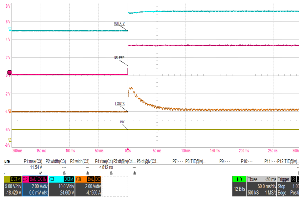
A. チャンネル 1 = IN1、 IN2 (並列) チャンネル 2 = V_{nSLEEP} チャンネル 3 = V_{OUT} (OUT1/2 の並列) チャンネル 8 = モーター 一電流
