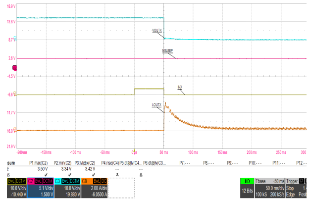
A. チャンネル 1 = IN1、 IN2 (並列) チャンネル 2 = V_{nSLEEP} チャンネル 3 = V_{OUT} (OUT1/2 の並列) チャンネル 8 = モーター 一電流
