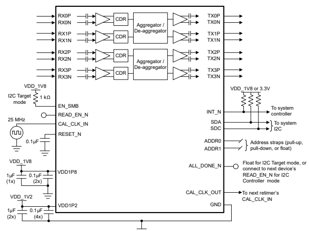
簡略回路図
