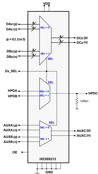
機能ブロック図
