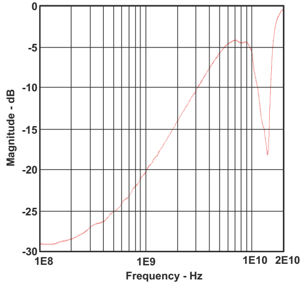
6-2. Return Loss
