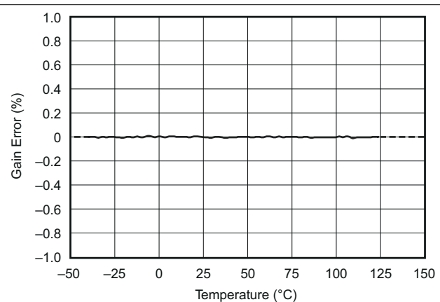
図 5-6. ゲイン誤差と温度との関係
