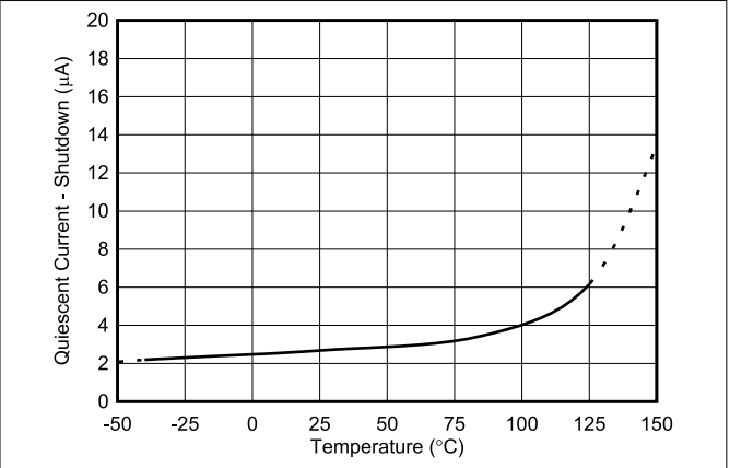
図 6-21. シャットダウン I_Q と温度の関係
