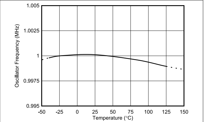
図 6-25. 内部クロック周波数と温度の関係
