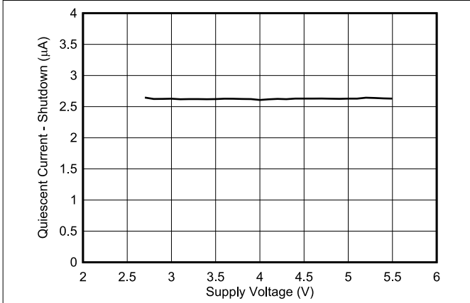
図 6-20. シャットダウン I_Q と電源電圧の関係
