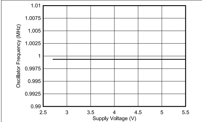
図 6-24. 内部クロック周波数と電源の関係
