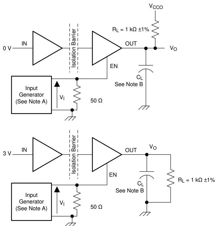
図 6-1. スwitching特性試験回路と電圧波形
