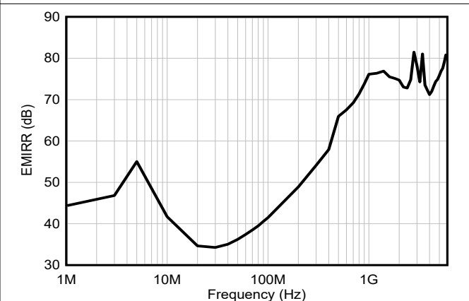
図 5-34. EMIRR (電磁干渉除去比) と周波数との関係
