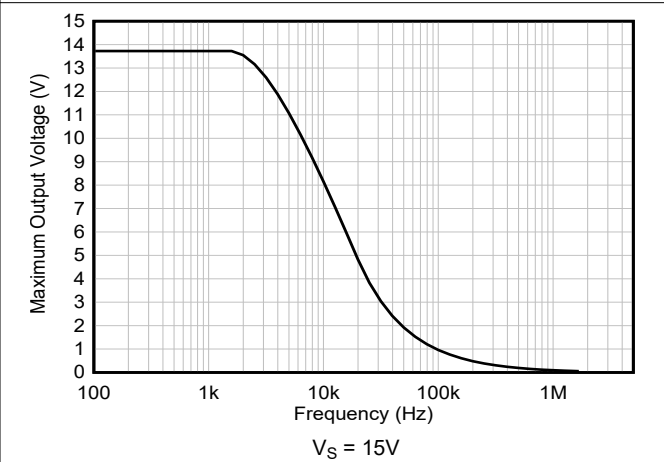
図 5-32. 最大出力電圧と周波数との関係 V_S = 15\text{V}
