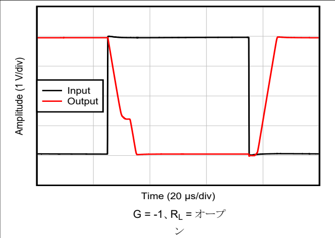
図 5-30. 大信号ステップ応答、 G = -1
