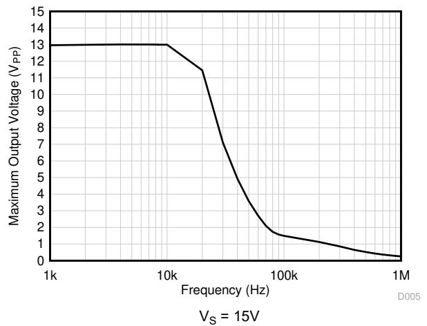
図 6-36. 最大出力電圧と周波数との関係
