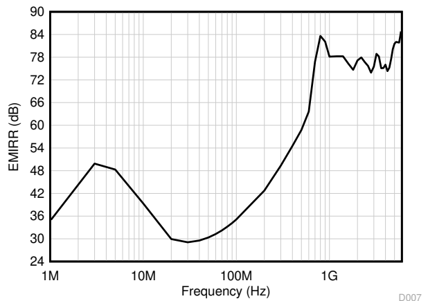
図 6-38. EMIRR (電磁干渉除去比) と周波数との関係
