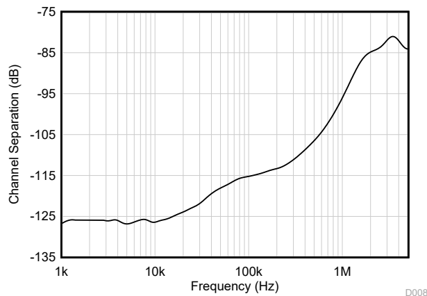
図 6-37. チャネル・セパレーションと周波数との関係
