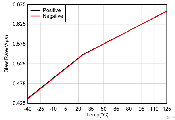
図 6-34. スルーレートと温度との関係
