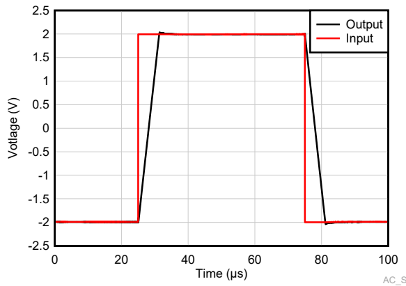
図 6-33. 大信号ステップ応答
