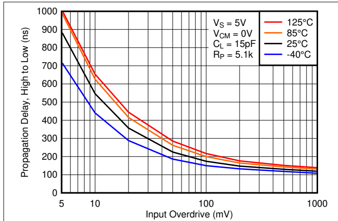
図 6-30. High から Low までの伝搬遅延と入力オーバードライブ電圧との関係、5V
