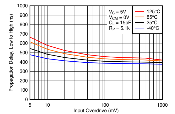
図 6-31. Low から High までの伝搬遅延と入力オーバードライブ電圧との関係、5V
