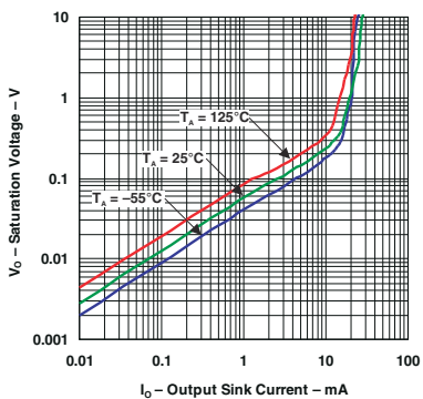
図 6-3. 出力飽和電圧
