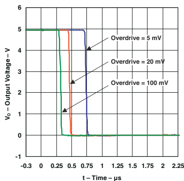
図 6-4. 各種オーバードライブの負の遷移に対する応答時間
