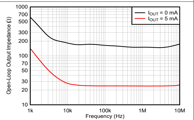
図 5-20. 開ループ出力インピーダンスと周波数との関係
