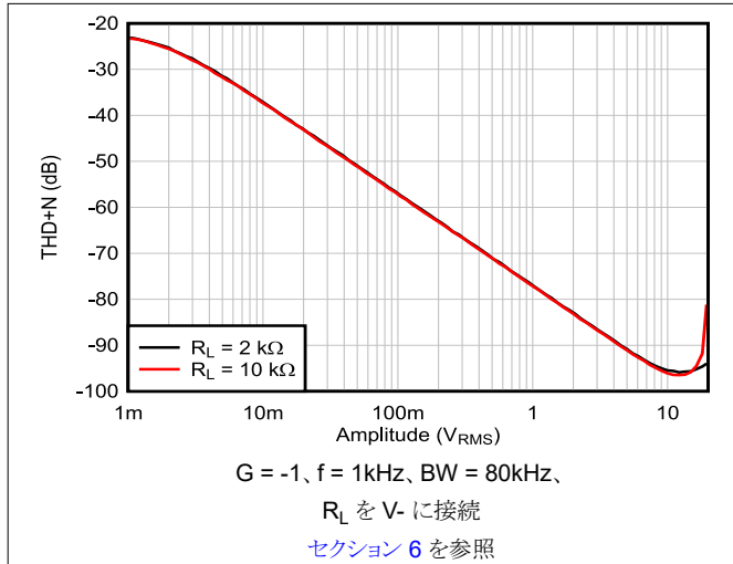
図 5-17. THD+N と出力振幅との関係、 G = -1
