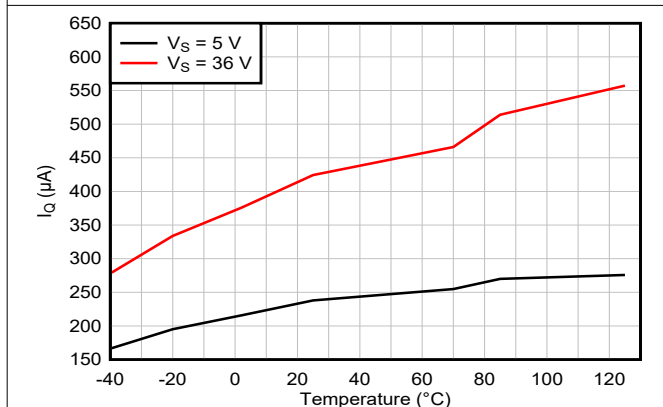
図 5-19. 静止電流と温度との関係
